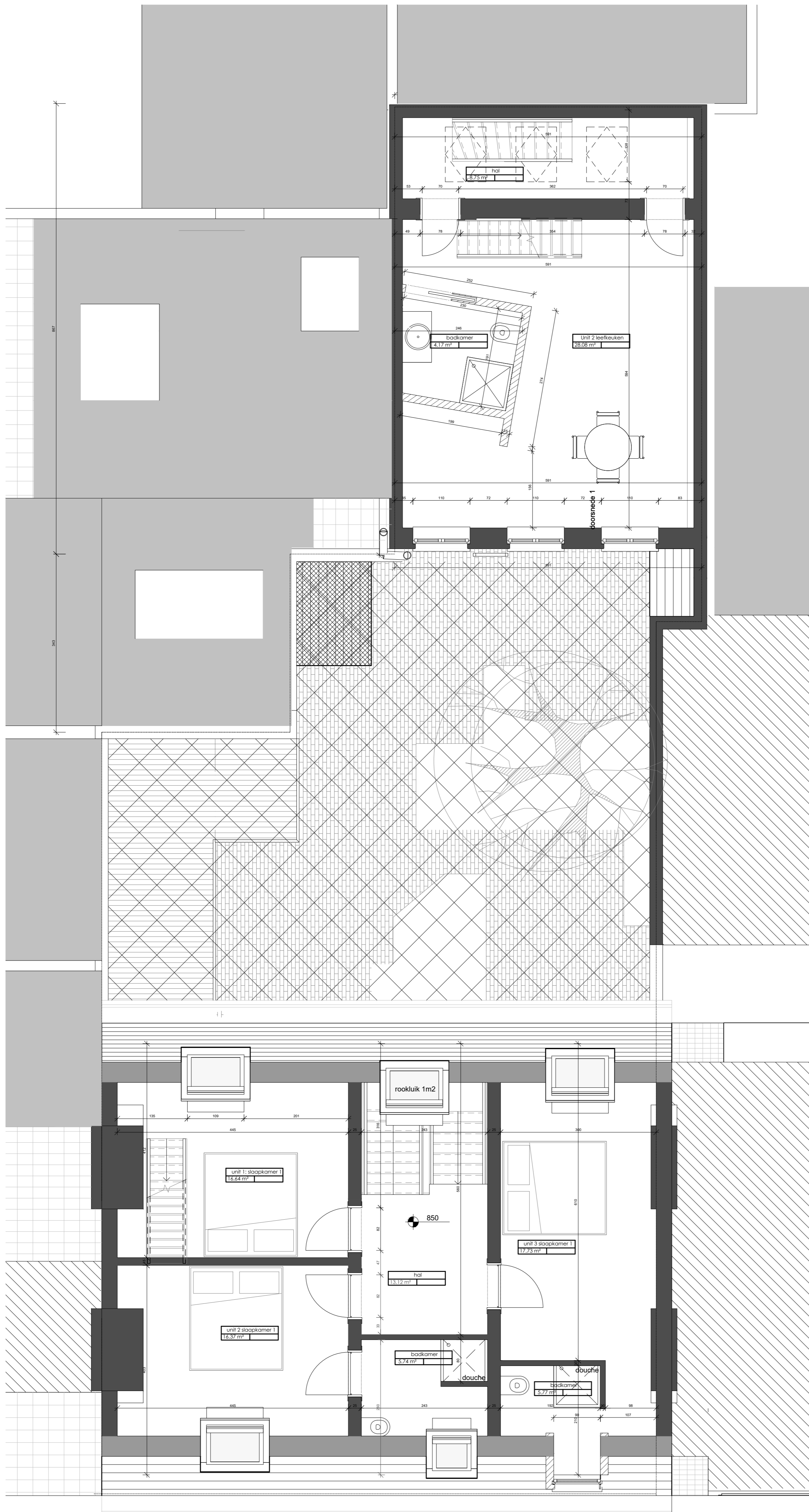
GRONDPLAN verdieping 2 bestaande toestand schaal: 1/100
