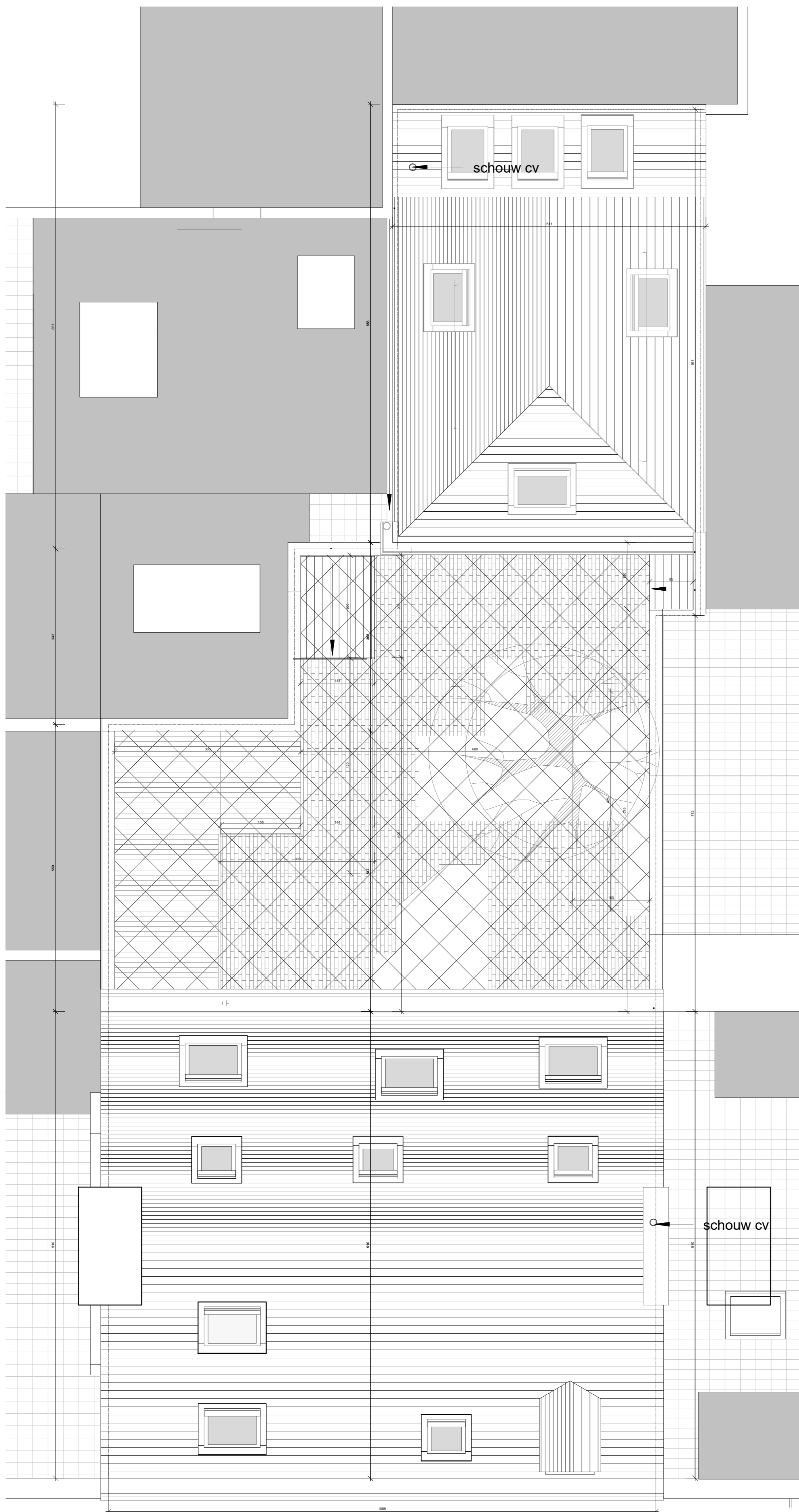
GRONDPLAN DAK bestaande toestand schaal: 1/100
