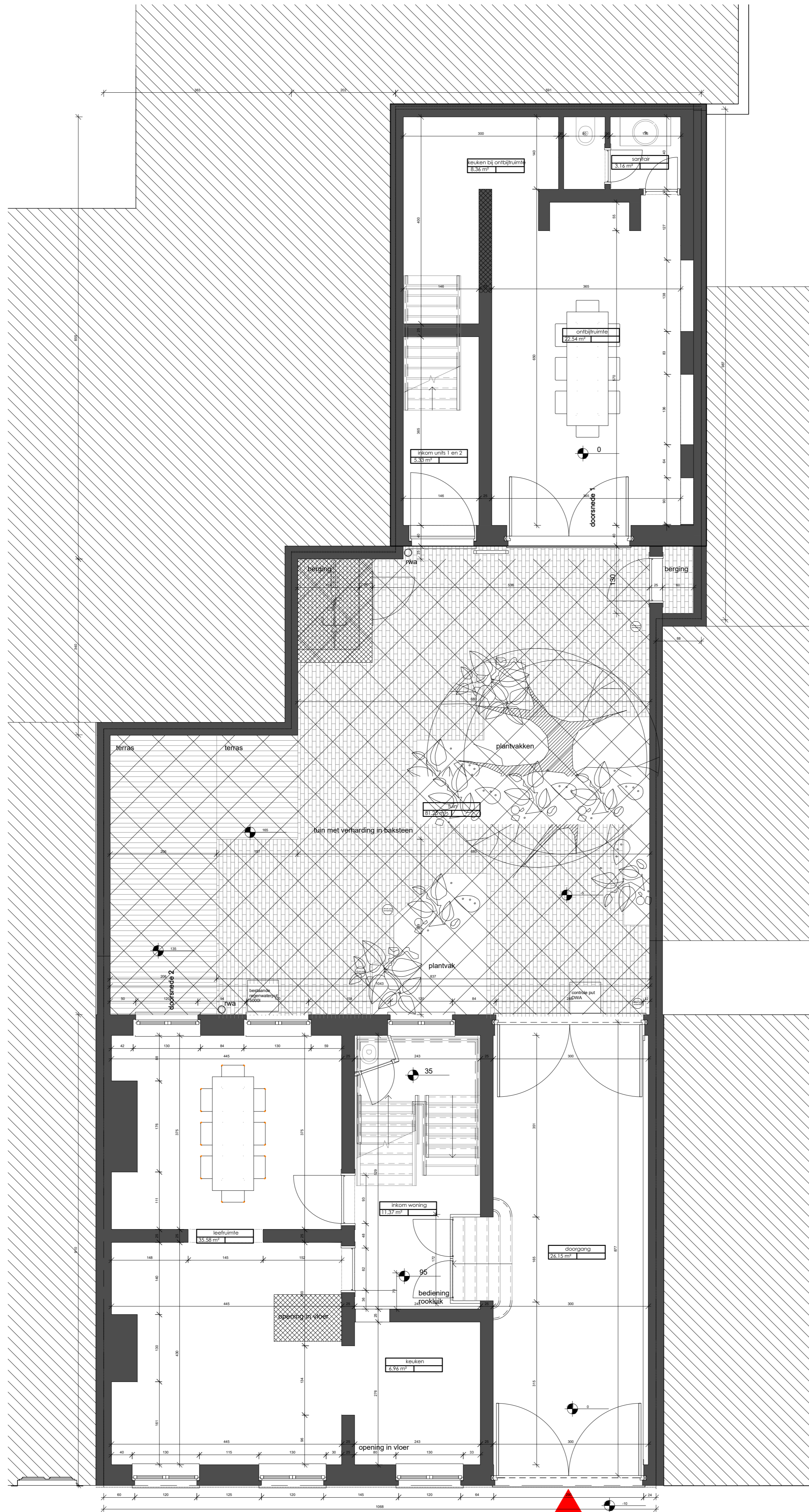
GRONDPLAN gelijkvloers bestaande toestand schaal: 1/100
