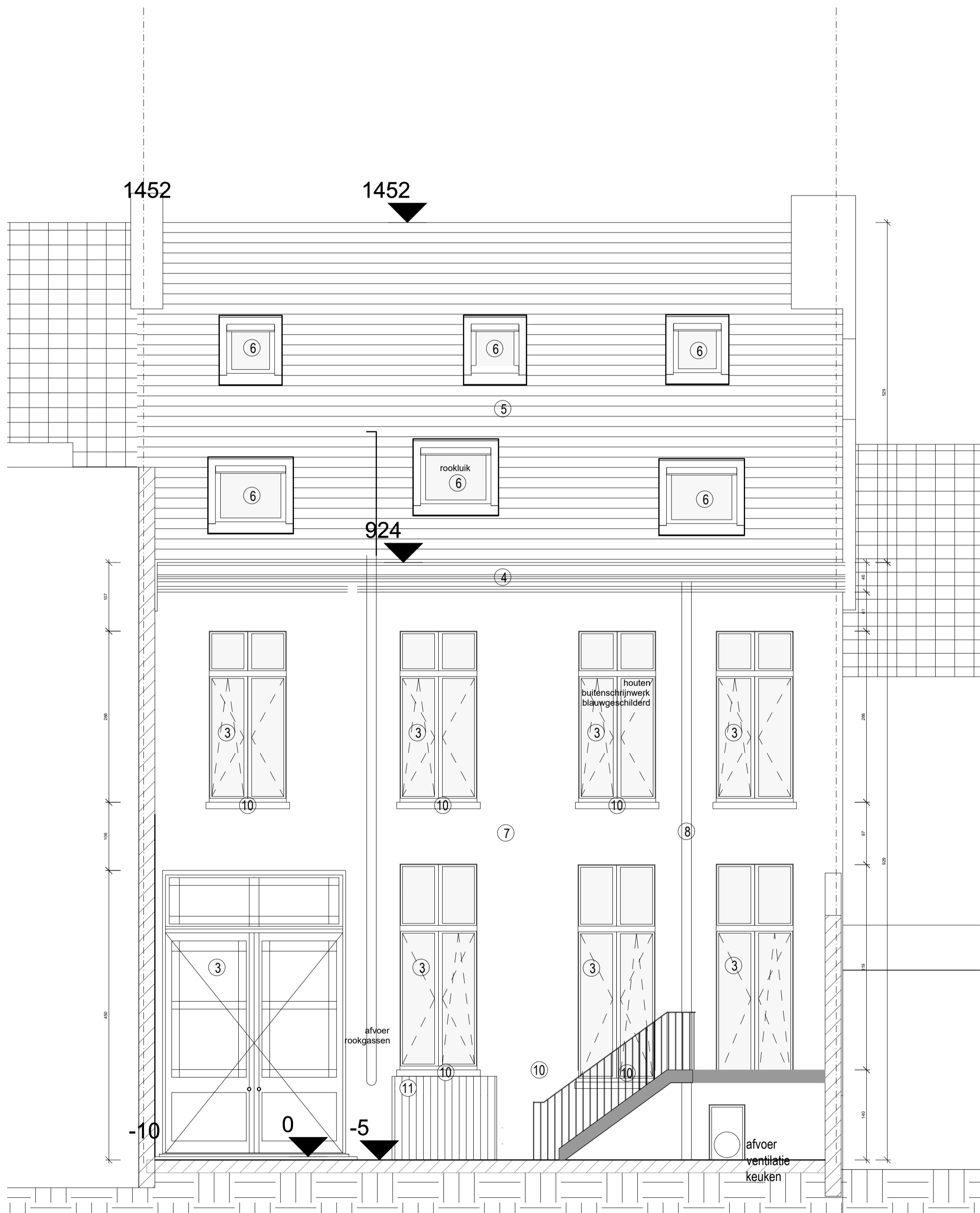
GEVEL 02: VOORHUIS nieuwe toestand schaal: 1/100
