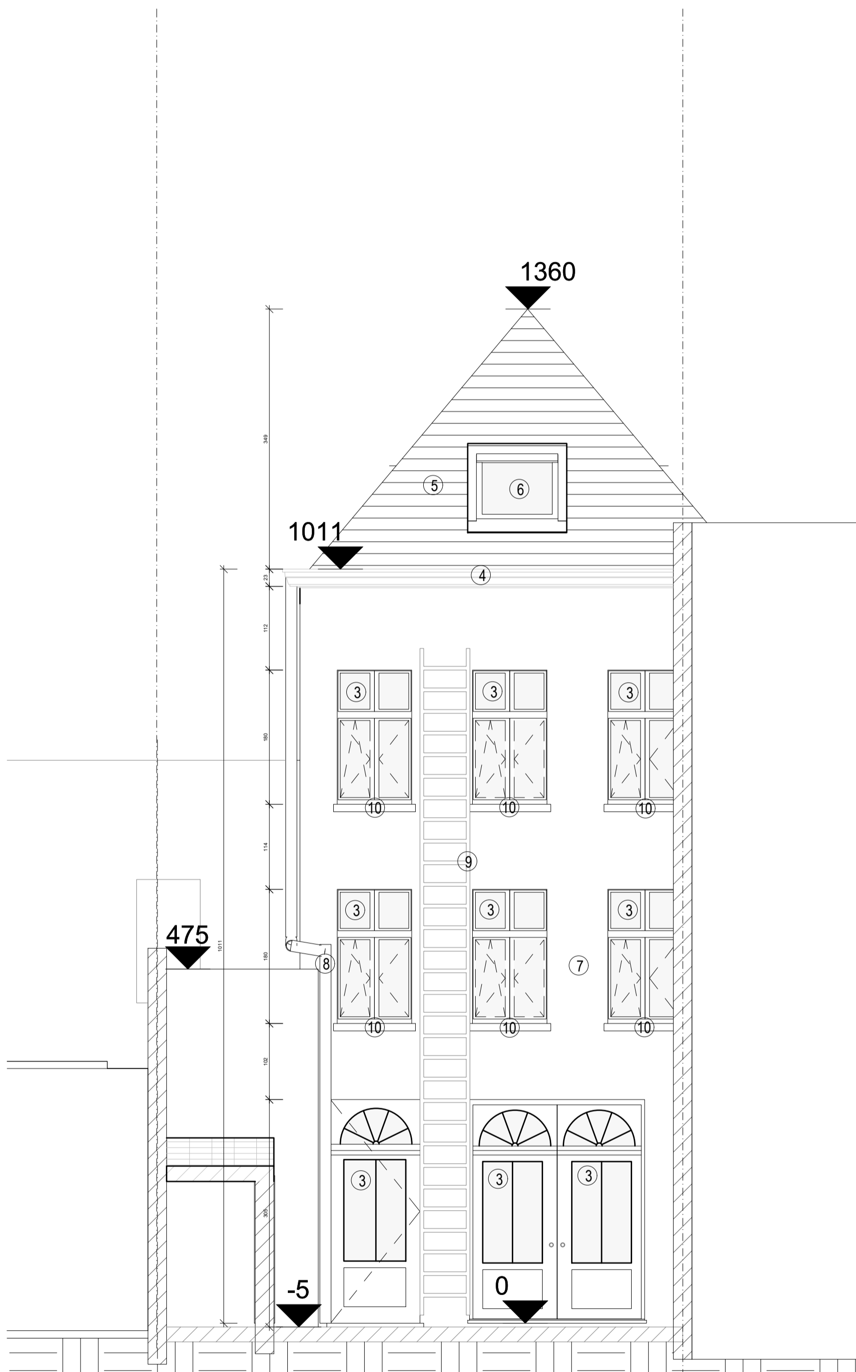
GEVEL 03: ACHTERHUIS nieuwe toestand schaal: 1/100
