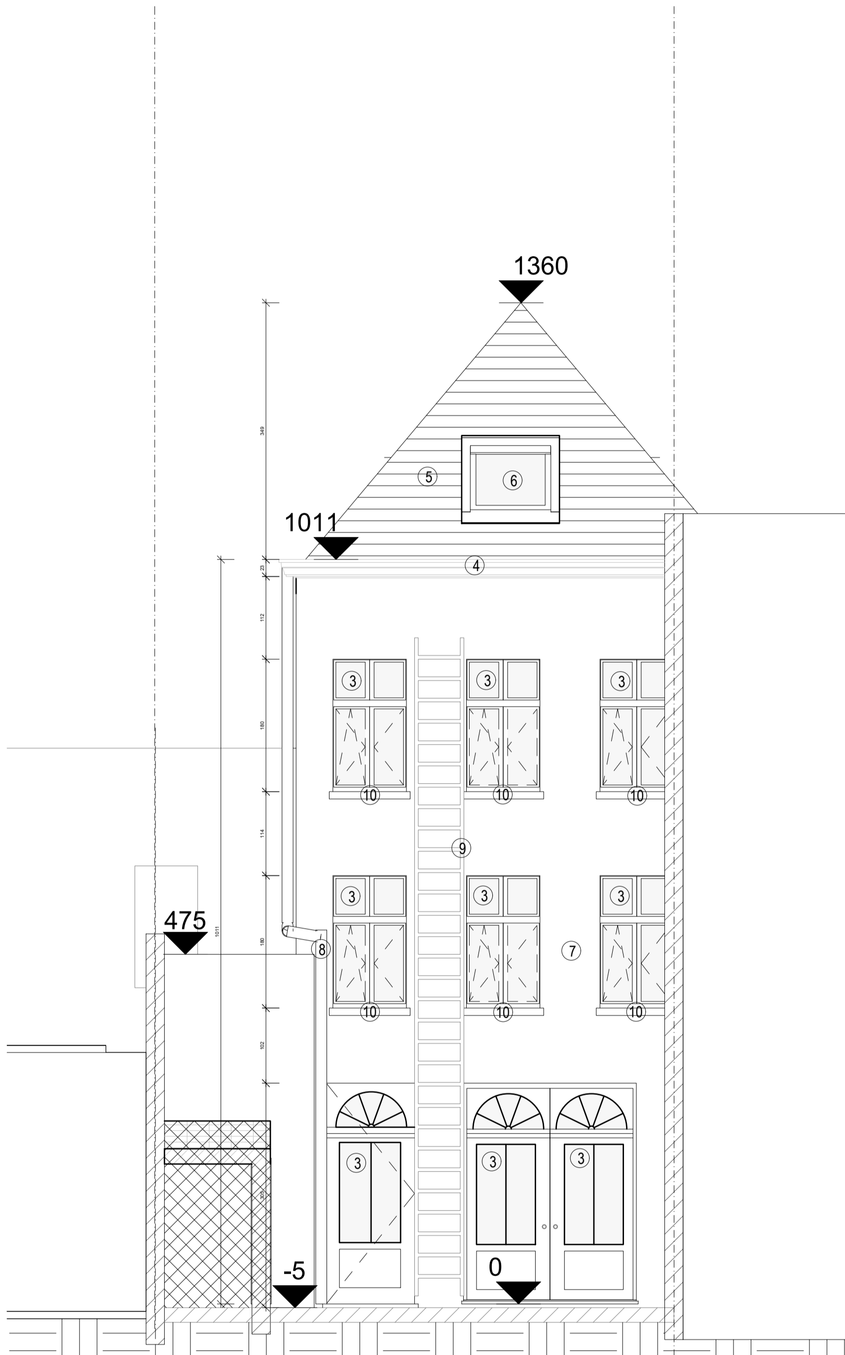
GEVEL 03: ACHTERHUIS bestaande toestand schaal: 1/100
