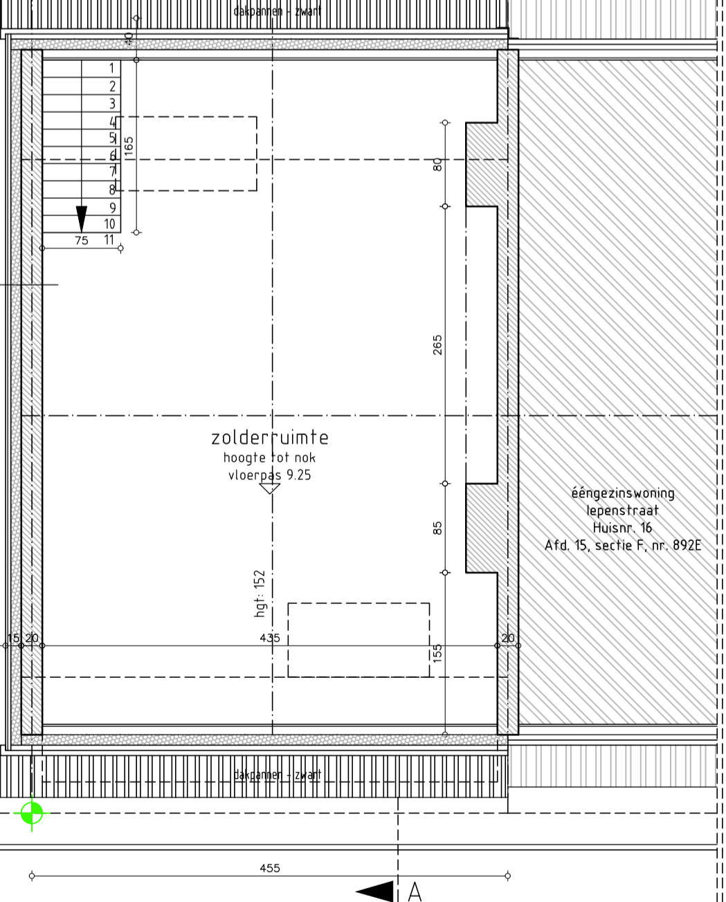
- Grondplan zolder - - Nieuwe toestand - - 1/50 -
