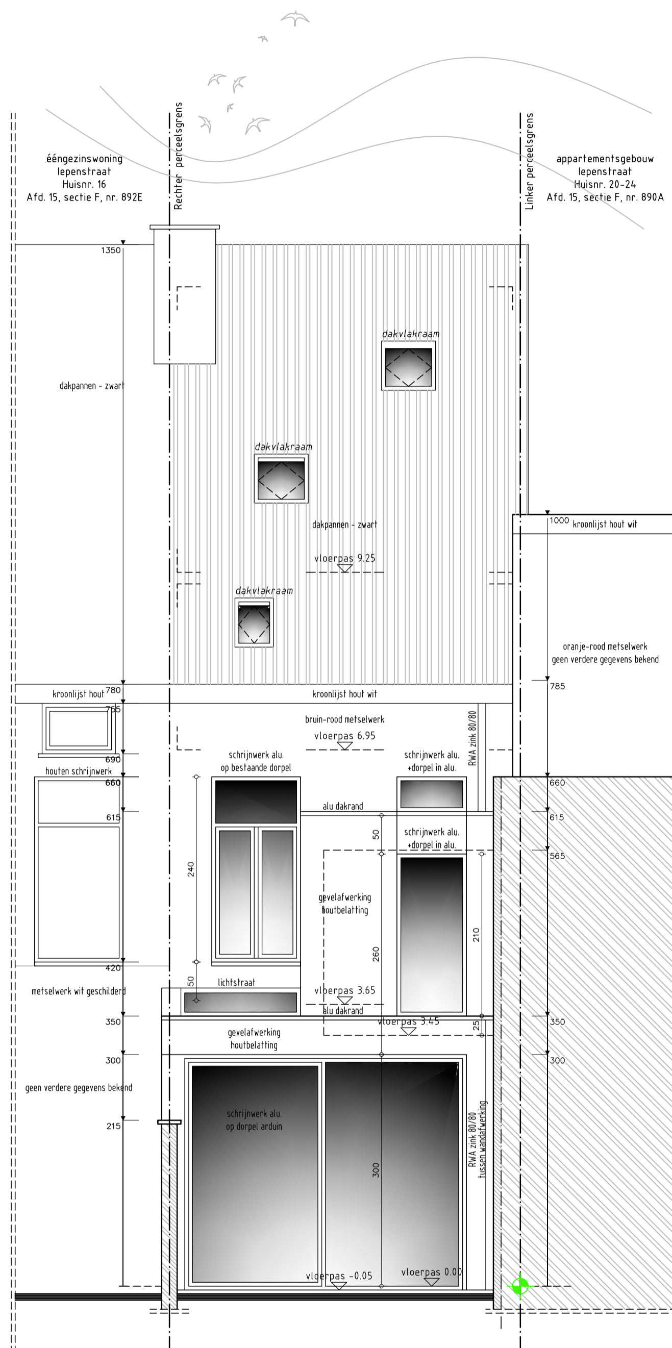
- Aanzicht achtergevel - - Bestaande toestand - - 1/50 -
