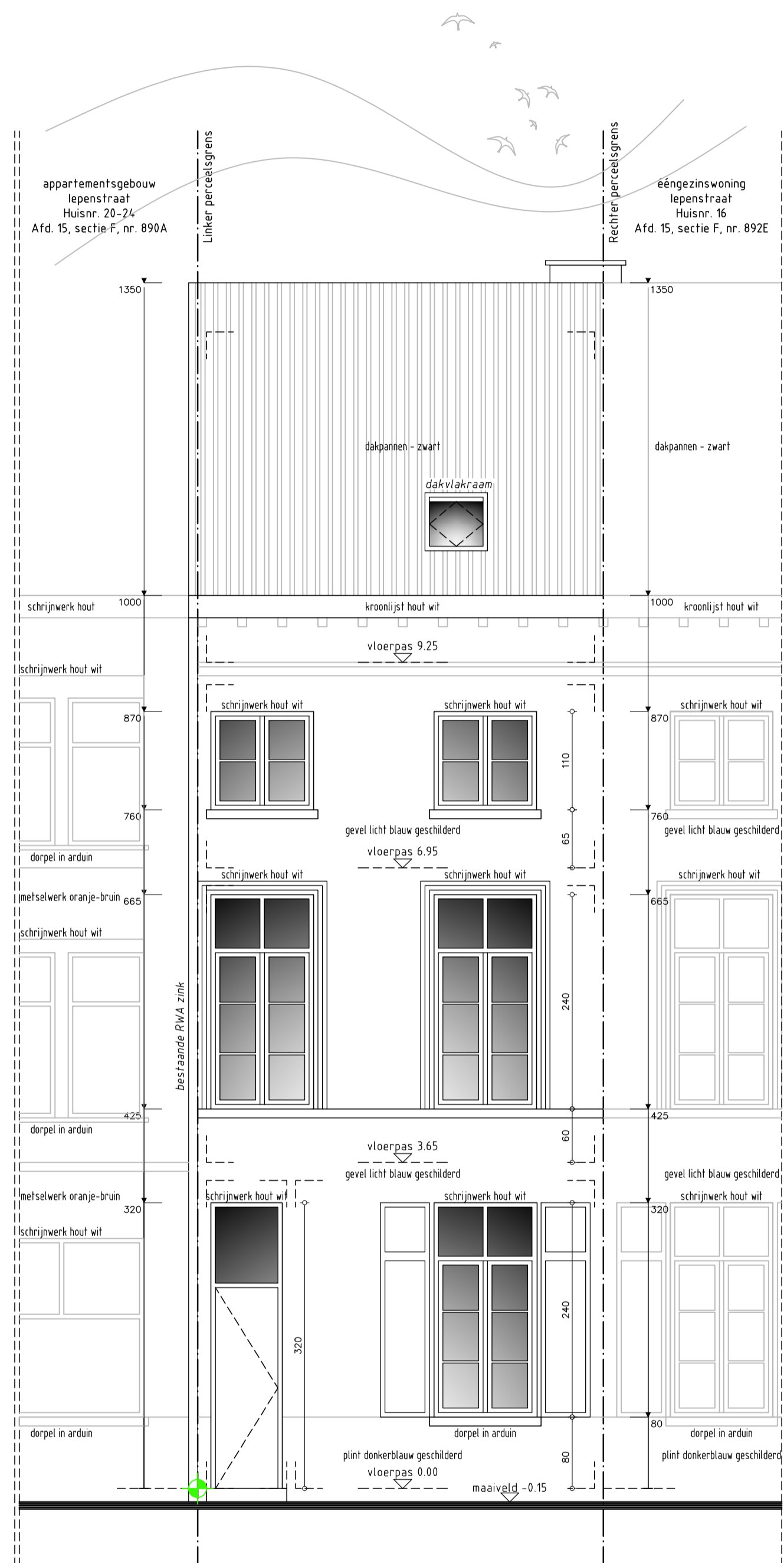
- Aanzicht voorgevel - - Bestaande toestand - - 1/50 -
