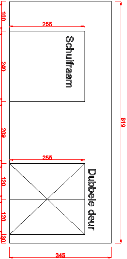
Zijaanzicht links
