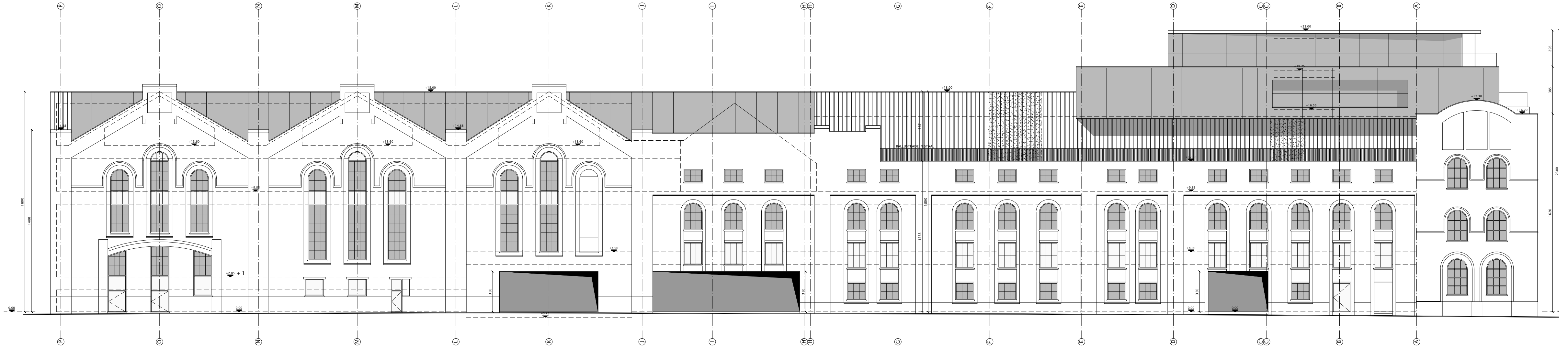
ZIJGEVEL LINKS (CARLSPLEIN) nieuwe toestand
