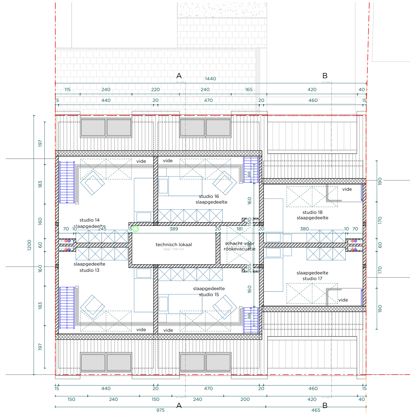
GRONDPLAN DERDE VERDIEPING (DUPLEXVERDIEPING)
