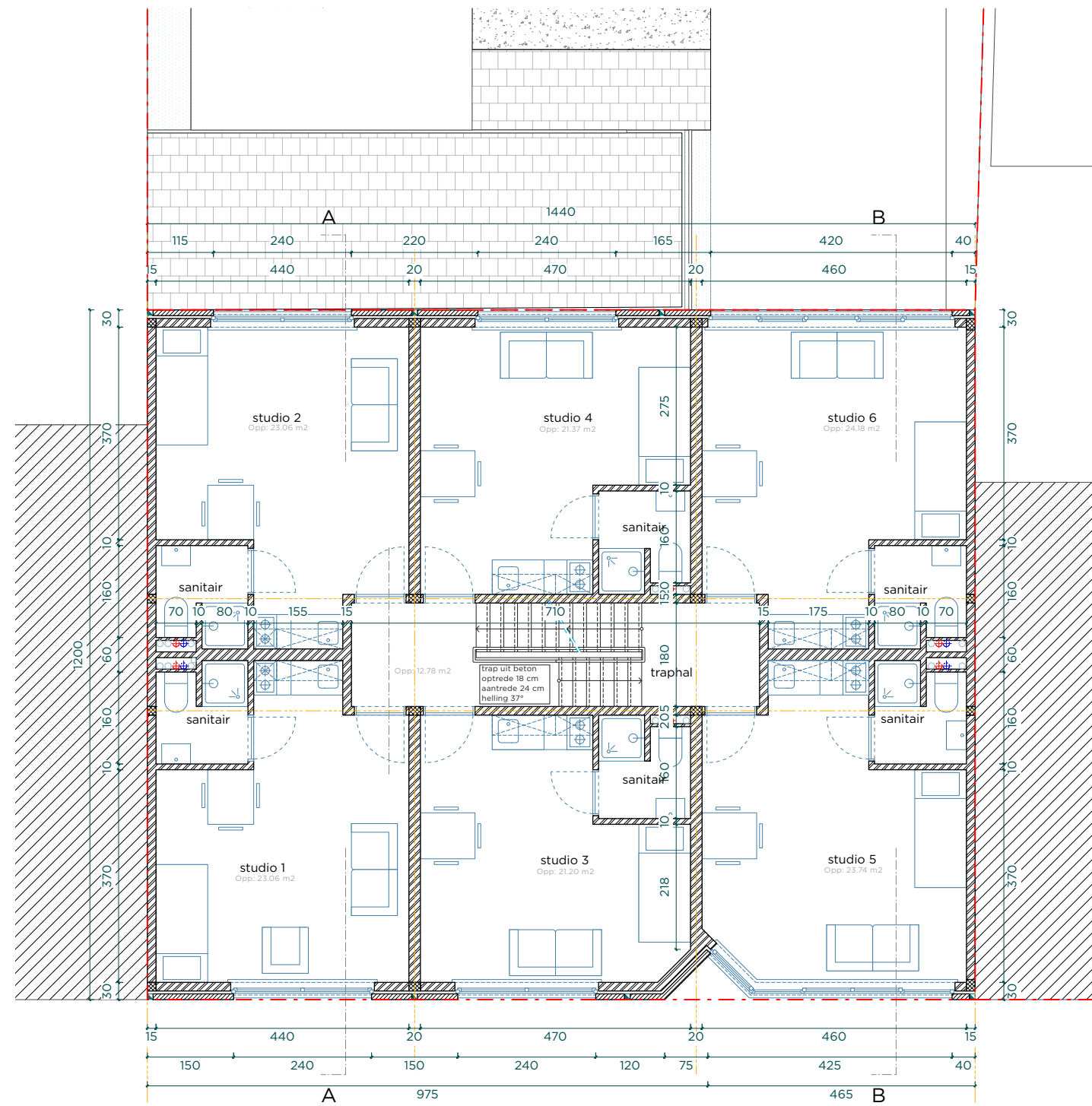
GRONDPLAN EERSTE VERDIEPING
