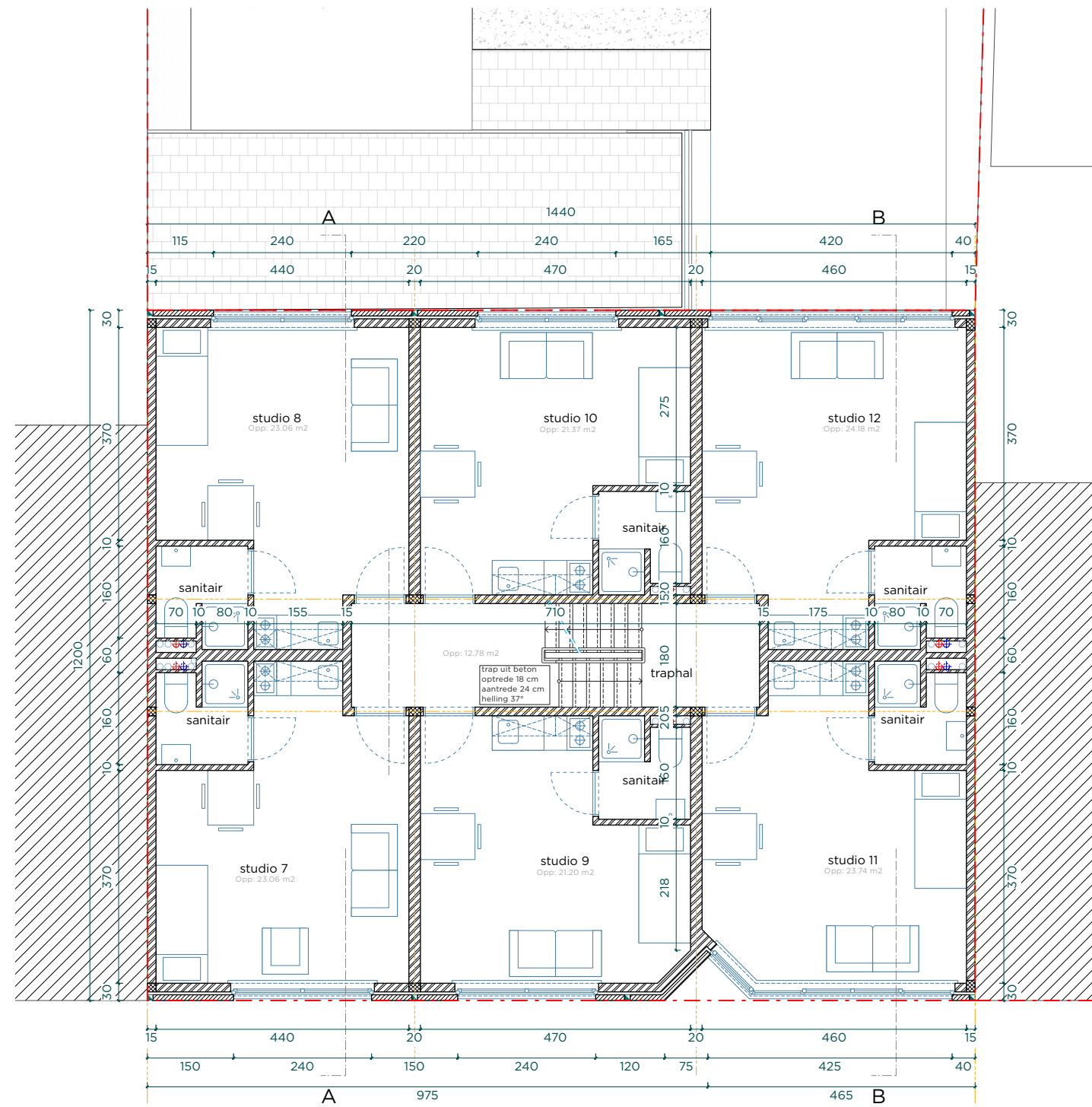
GRONDPLAN TWEEDE VERDIEPING
