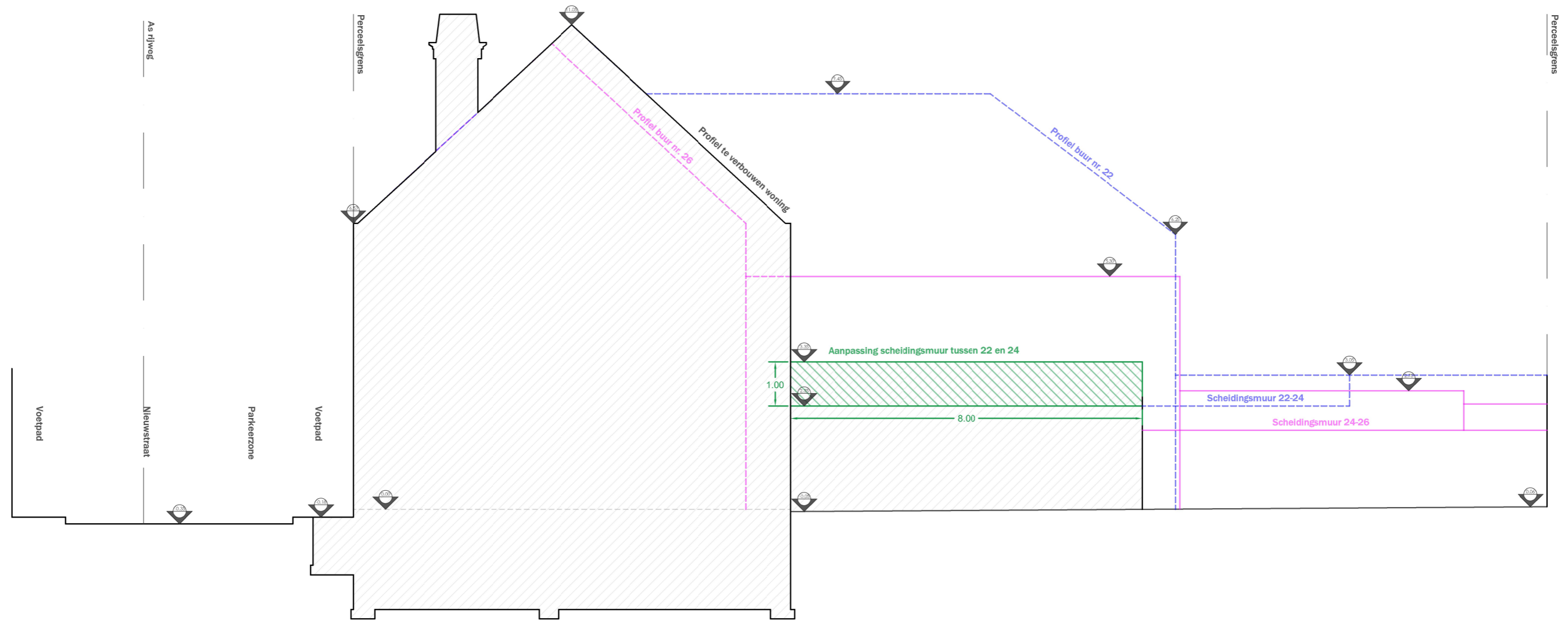
T TERREIN PROFIEL NIEUWE TOESTAND SCHAAAL: 1:100
