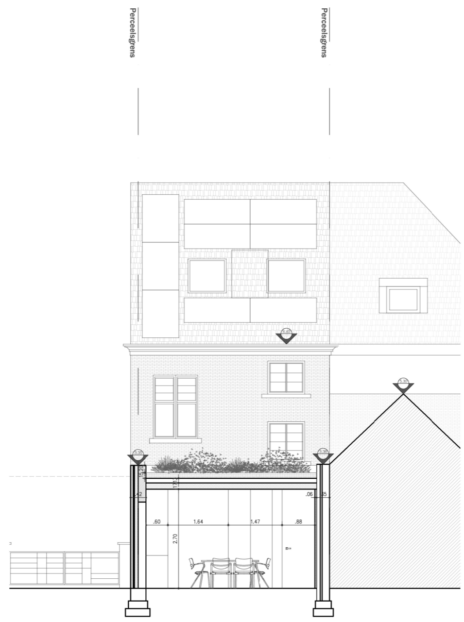
AA SNEDE AA' NIEUWE TOESTAND SCALE: 1/100
