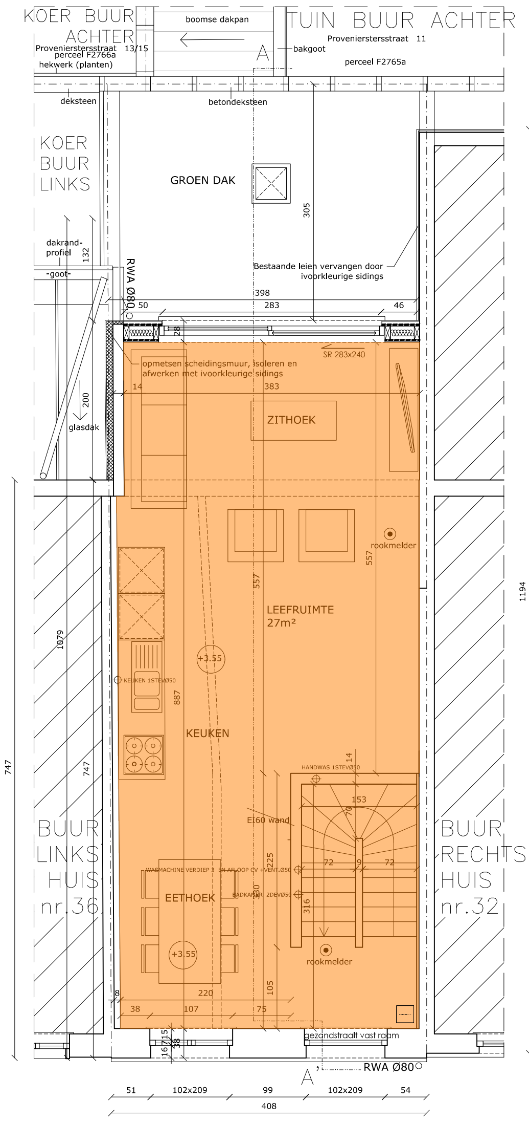
PLAN NR. 34 NIVEAU + 1
