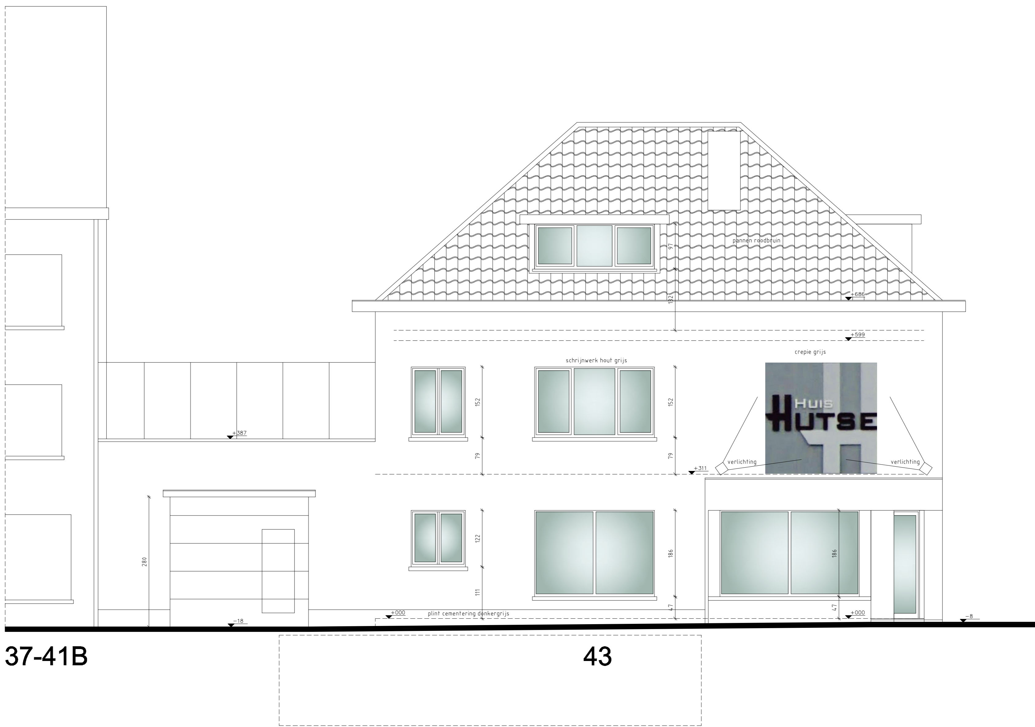
aanzicht voorgevel bestaande toestand 1/50
