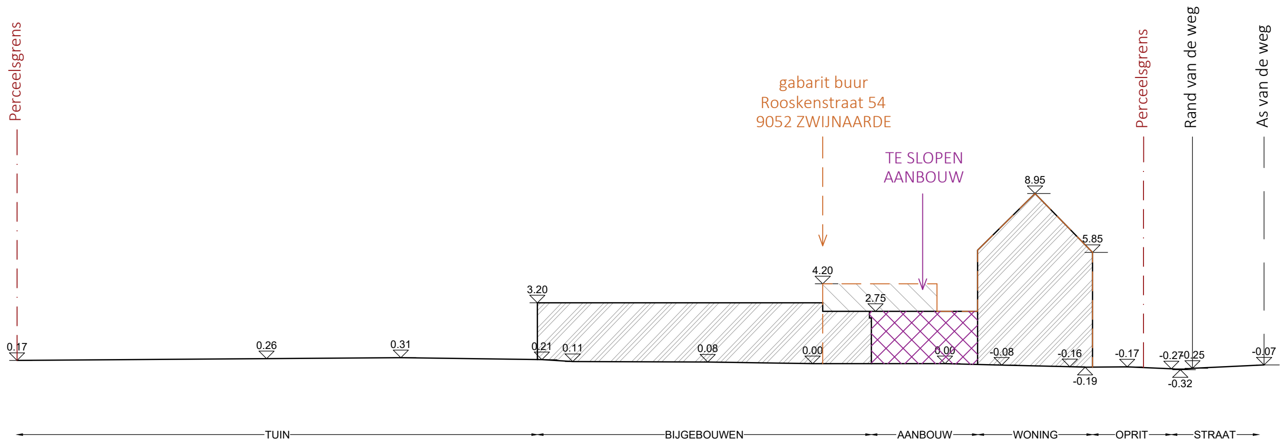
TERREINPROFIEL A bestaande toestand (= vergunde toestand)
