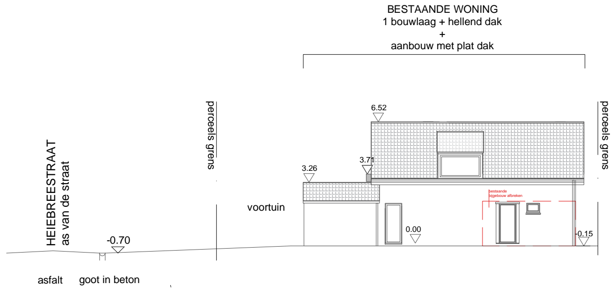
TERREINDOORSNEDE Bestaande toestand Schaal 1/200
