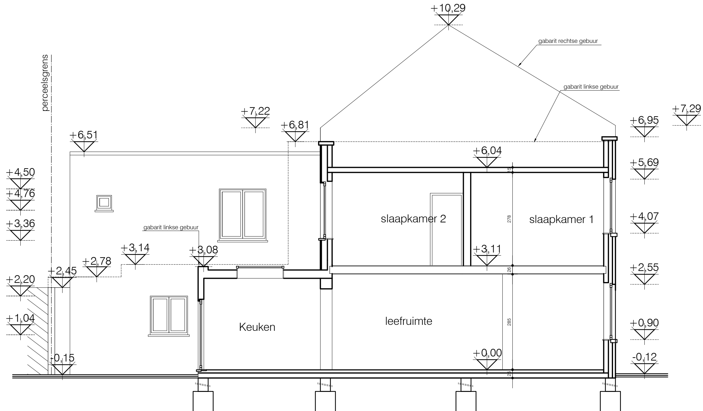
DOORSNEDE A-B Bestaande toestand alle afmetingen zijn in cm schaal 1/50
