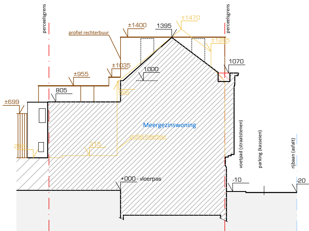
TERREINPROFIEL BESTAAND (sch. 1/200)
