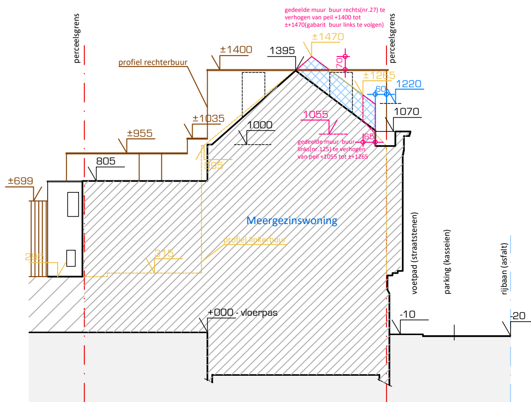
TERREINPROFIEL NIEUW (sch. 1/200)
