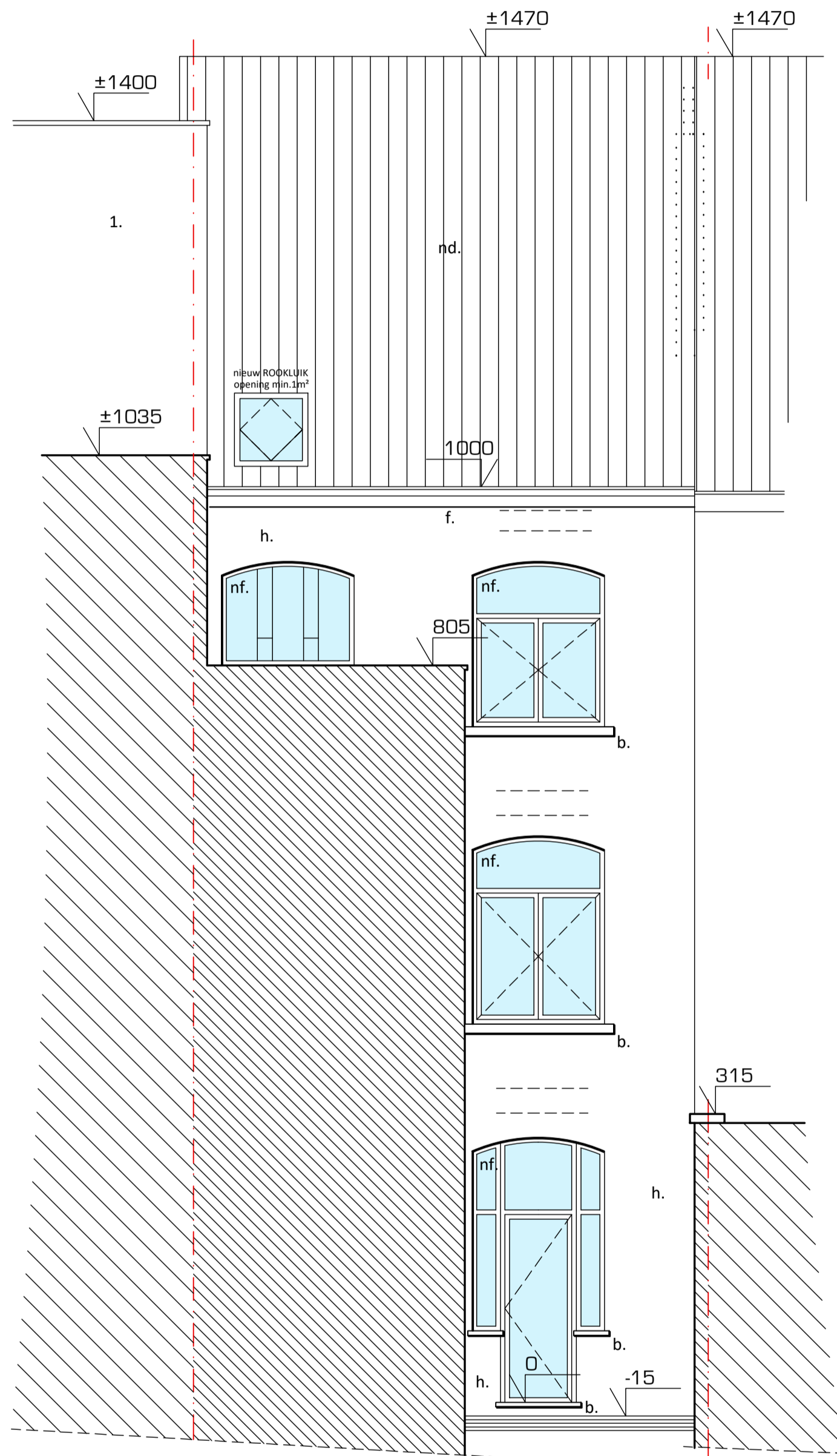
ACHTERGEVEL HOOFDGEBOUW
