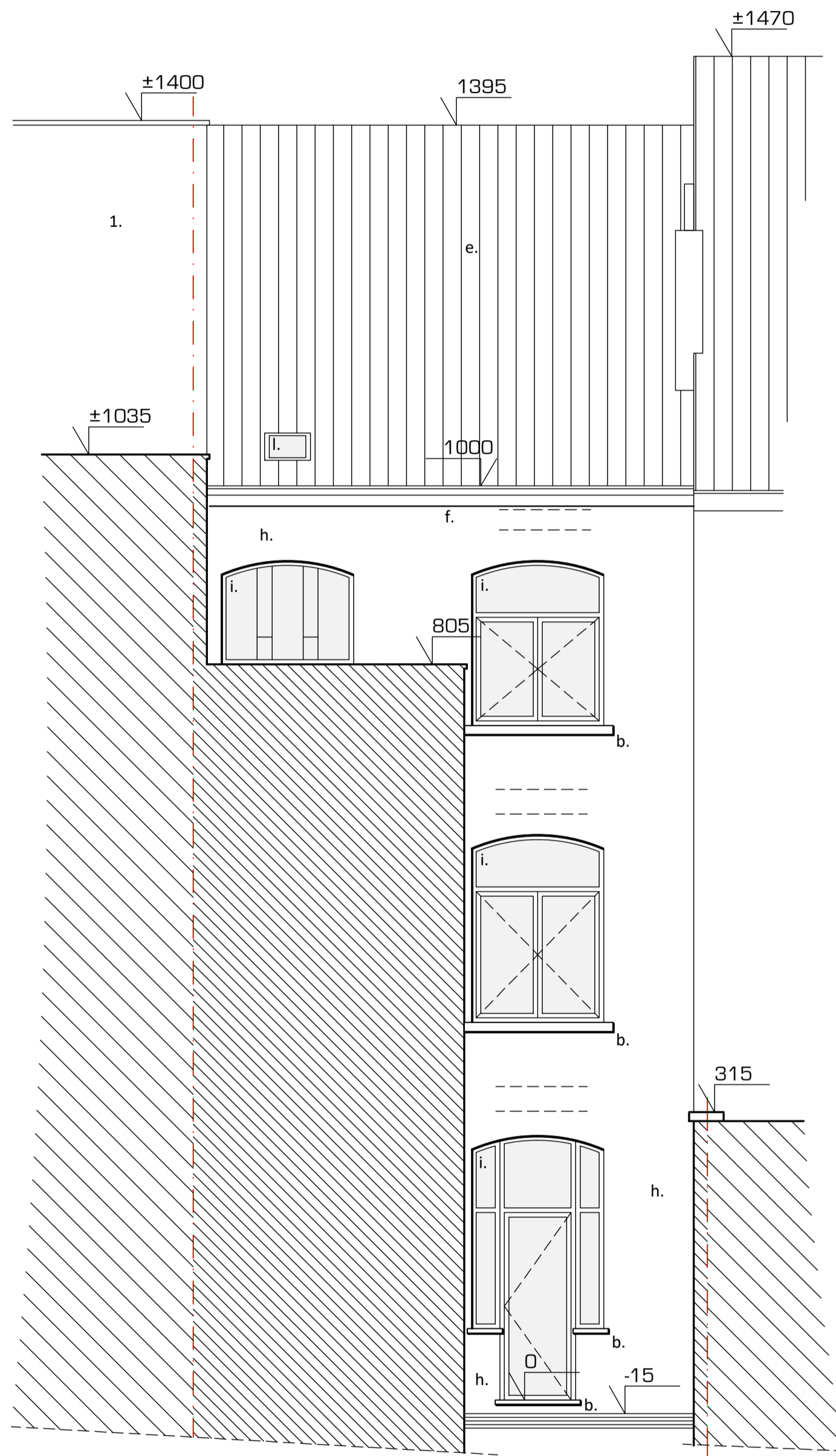
ACHTERGEVEL HOOFDGEBOUW
