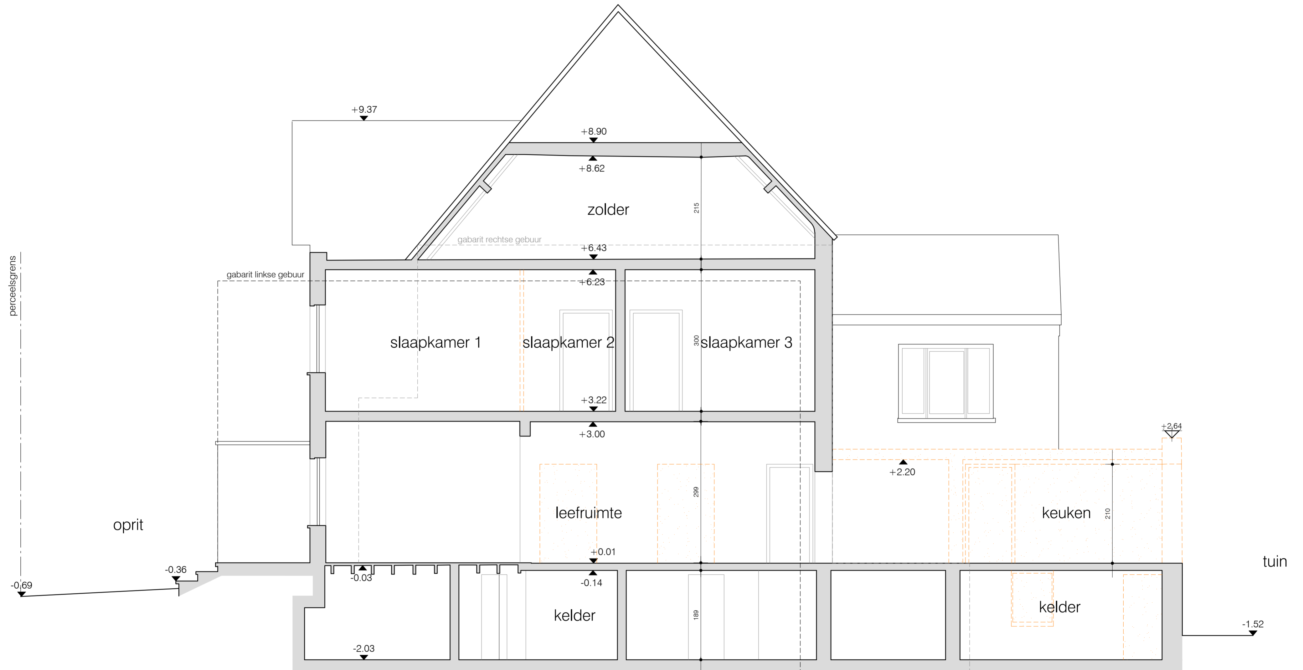
DOORSNEDE A-A Bestaande toestand alle afmetingen zijn in cm
