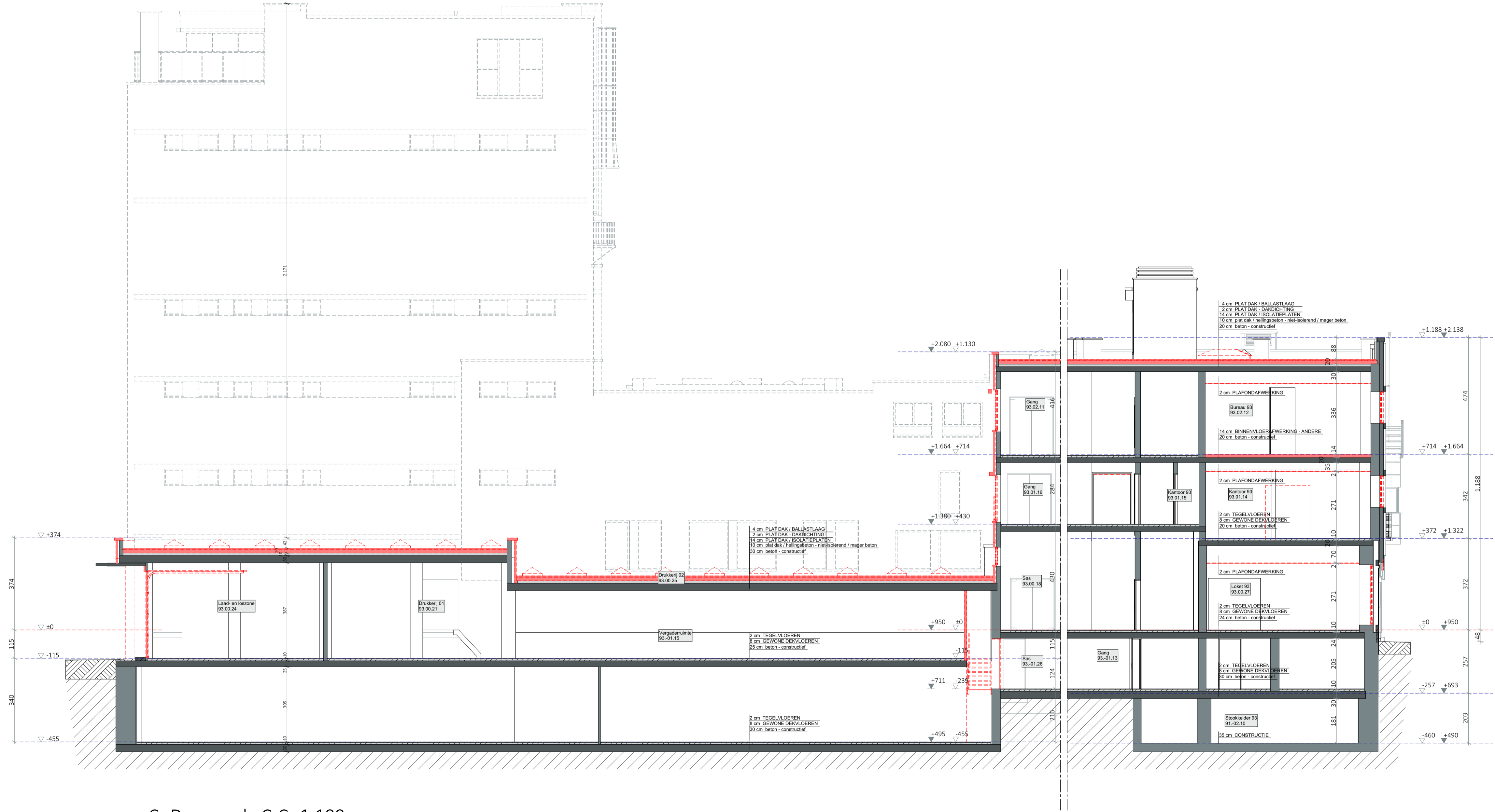
C- Doorsnede C-C- 1:100
