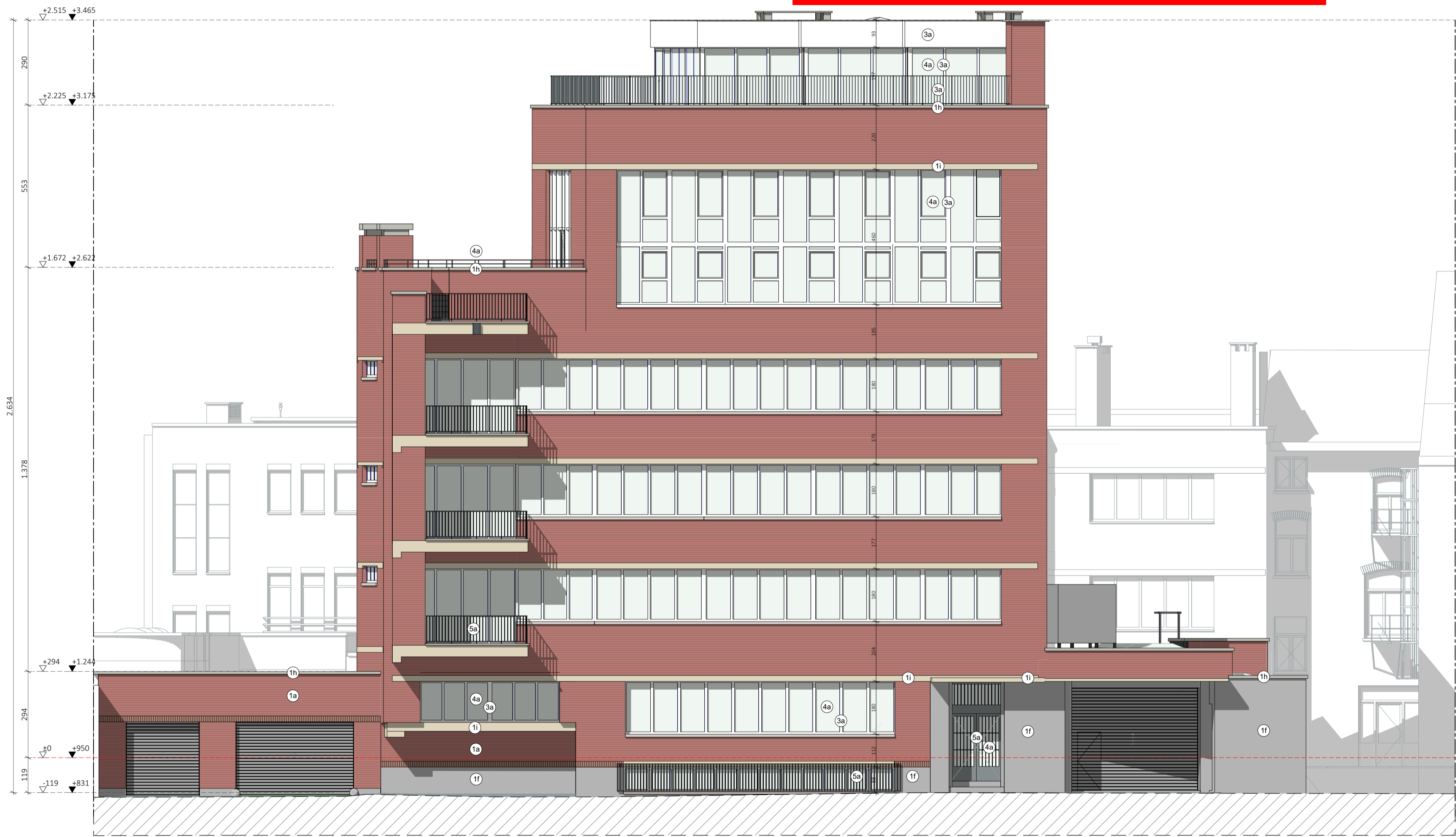
G5- Gevel 5- 1:100
