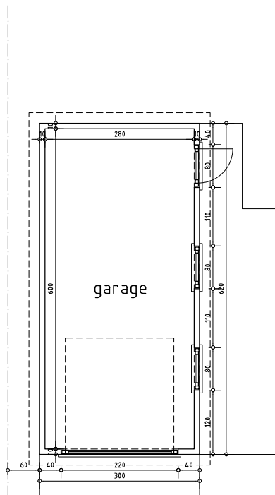
Grondplan – garage (bestaand)
