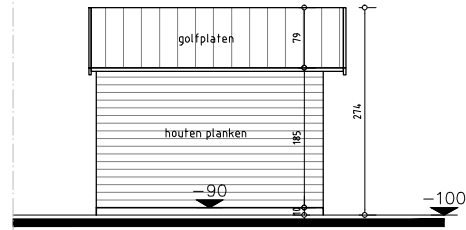
Voorgevel – tuinberging
