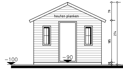
Gevel Rechts – tuinberging
