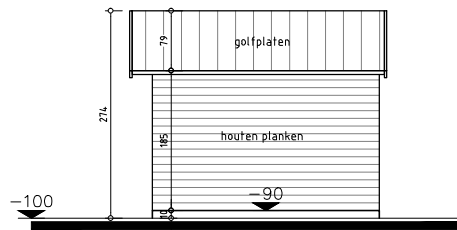
Achtergevel – tuinberging
