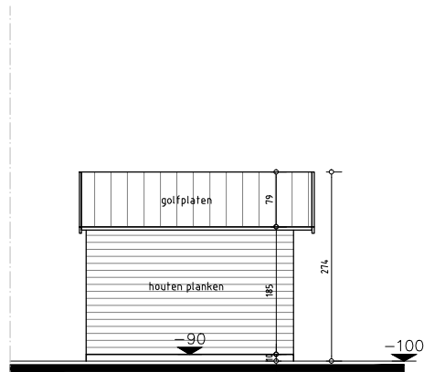
Voorgevel – tuinberging
