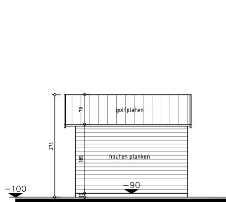
Achtergevel – tuinberging
