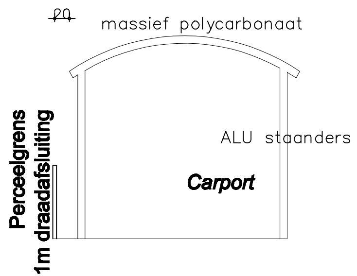
Achtergevel schaal 1/50
