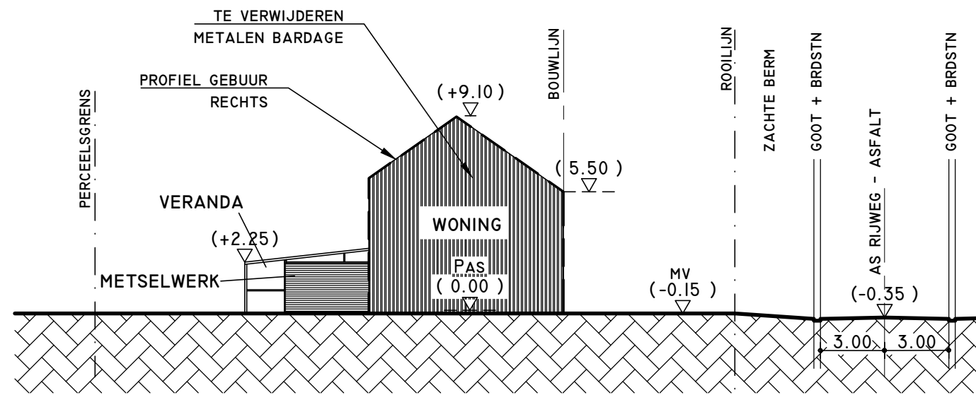
BESTAAND TERREINPROFIEL T-T
