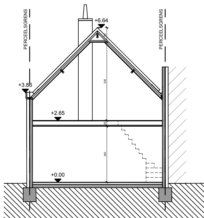
SNEDE B-B' / 1:100
