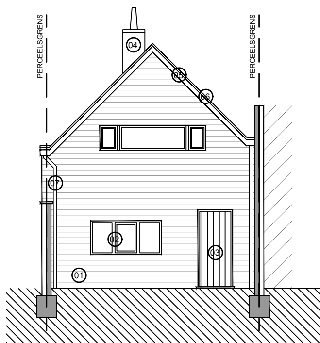
VOORGEVEL / 1:100
