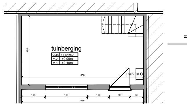
VLOERPLAN NIVEAU 0 / 1:100
