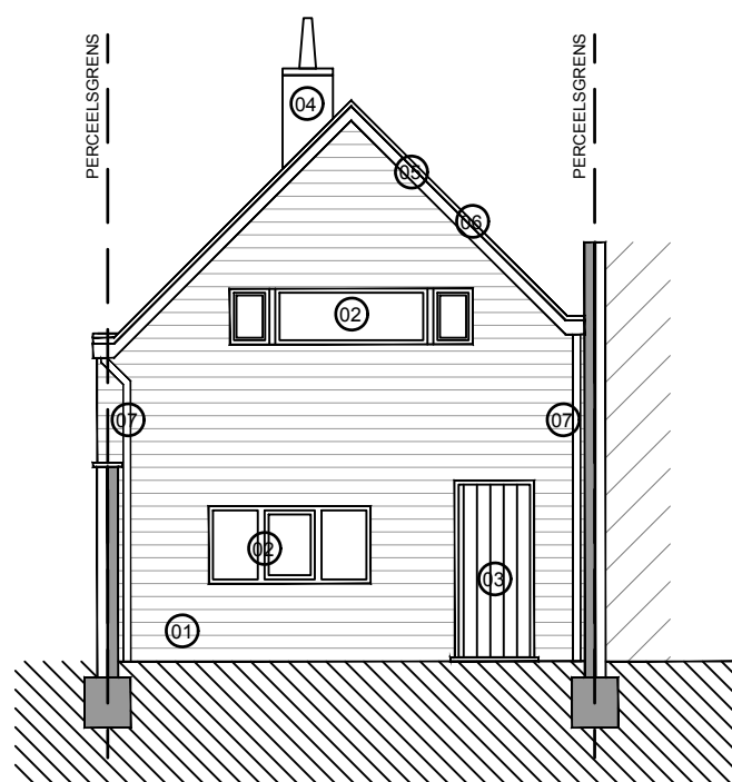
VOORGEVEL / 1:100
