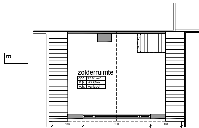
VLOERPLAN NIVEAU +1 / 1:100
