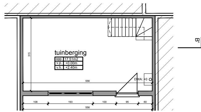
VLOERPLAN NIVEAU 0 / 1:100
