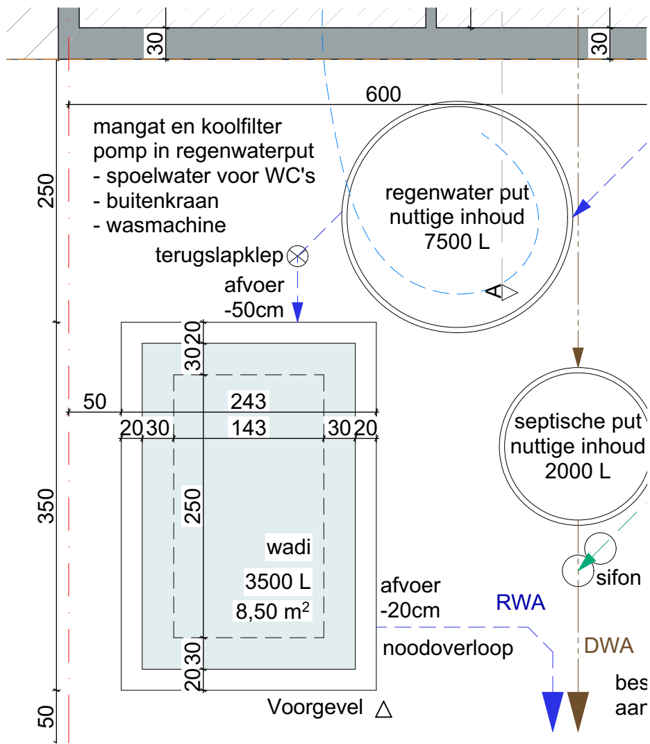
GRONDPLAN
