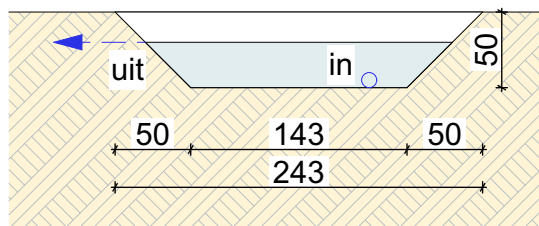
DWARSDOORSNEDE
