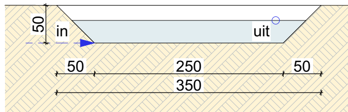
LANGSDOORSNEDE
