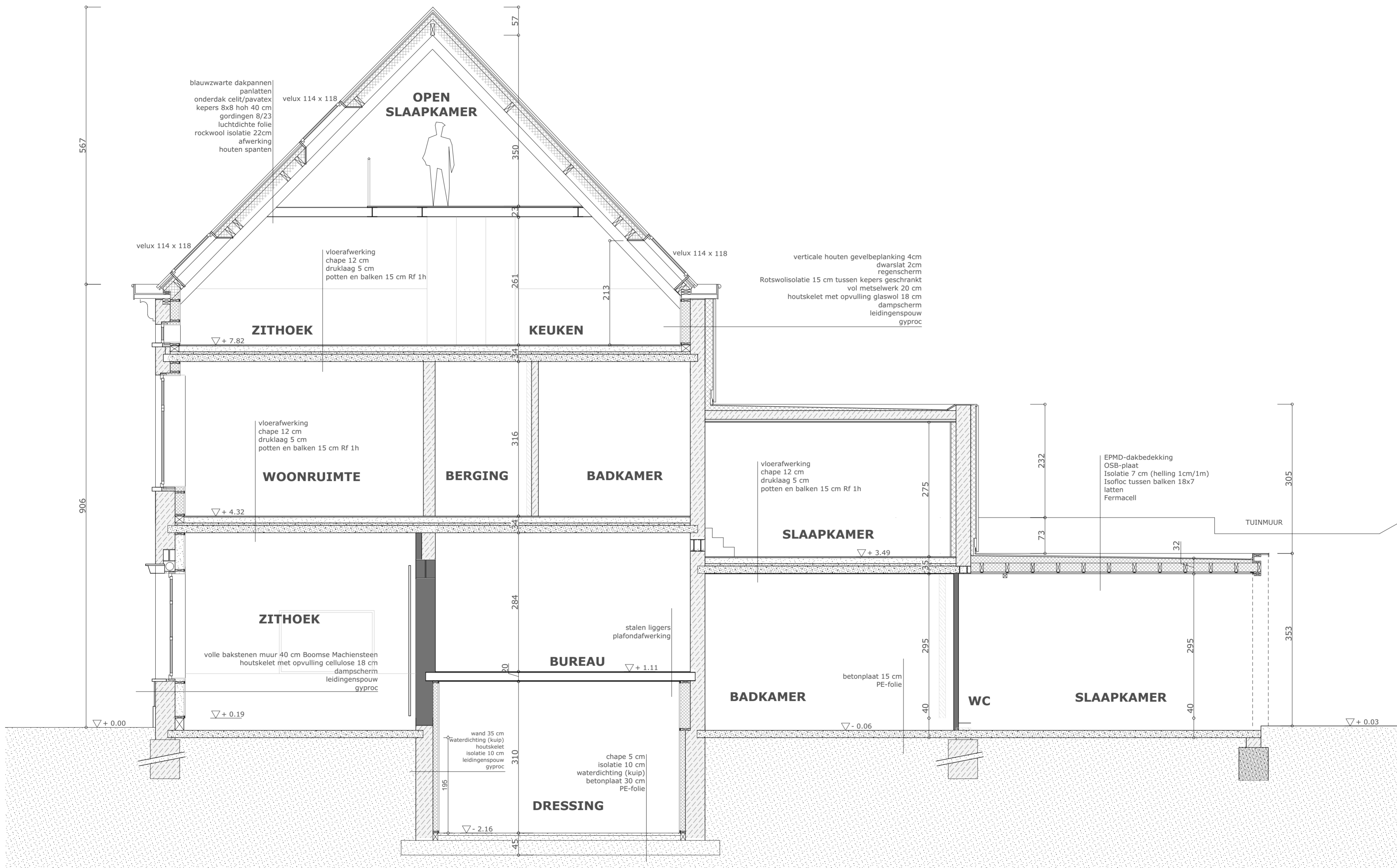
SNEDE CD bestaande toestand - schaal 1:50
