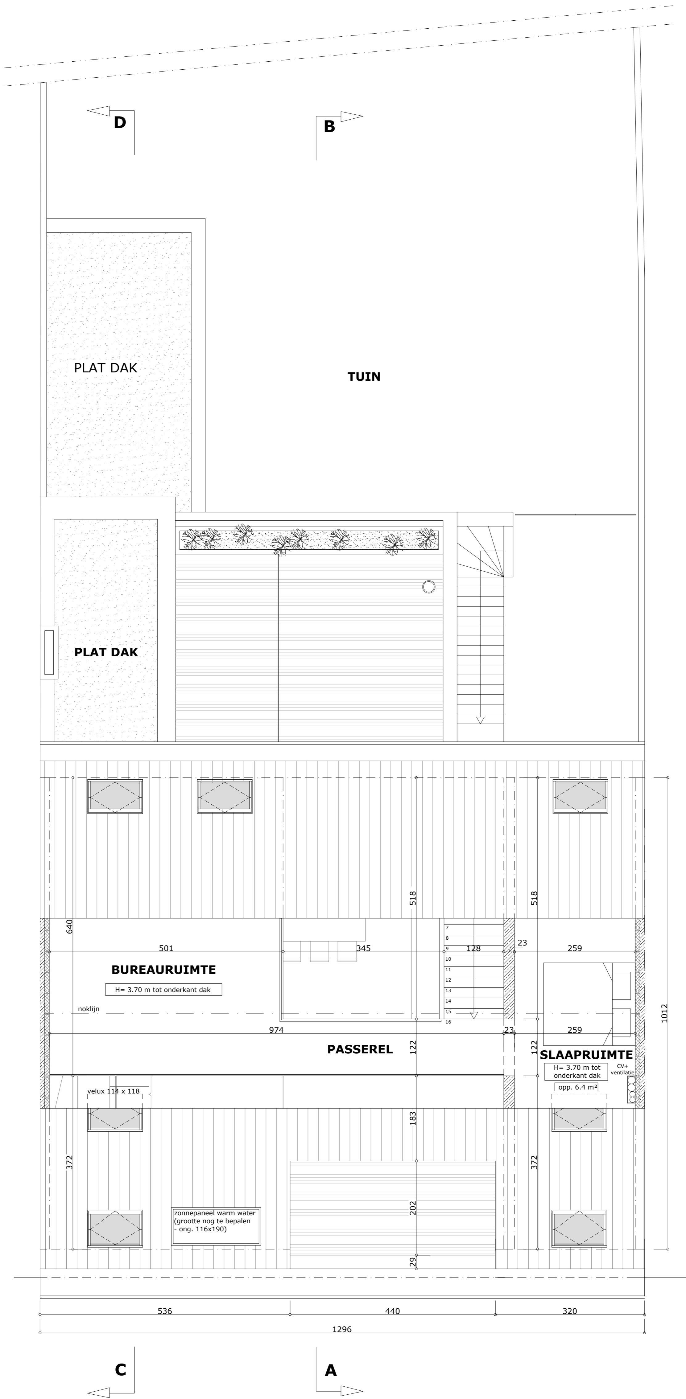
PLAN ZOLDER VERD. 2 vergunde toestand SCHAAL 1/50
