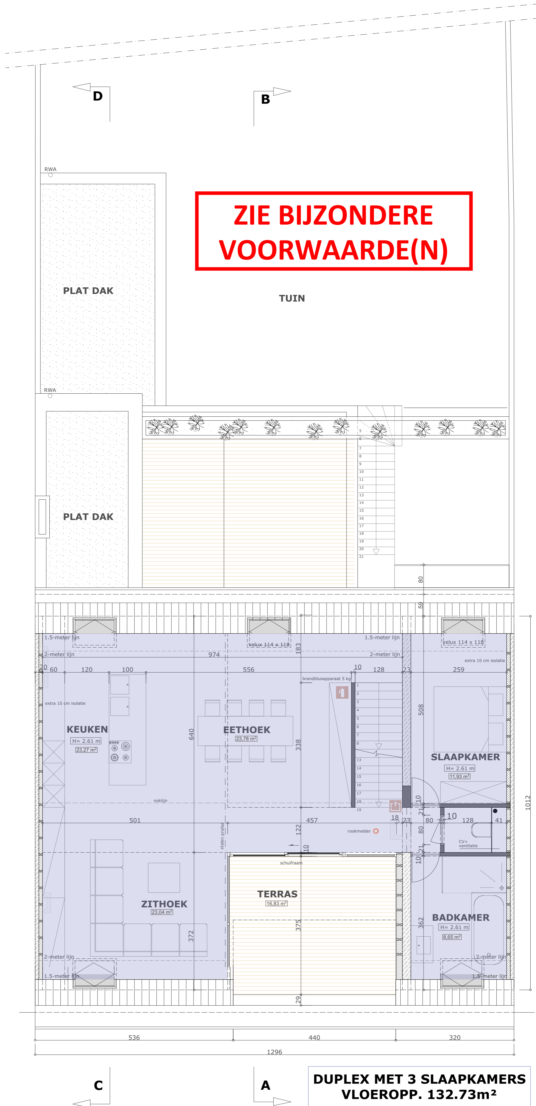
PLAN ZOLDER VERD. 1 nieuwe toestand - schaal 1:50
