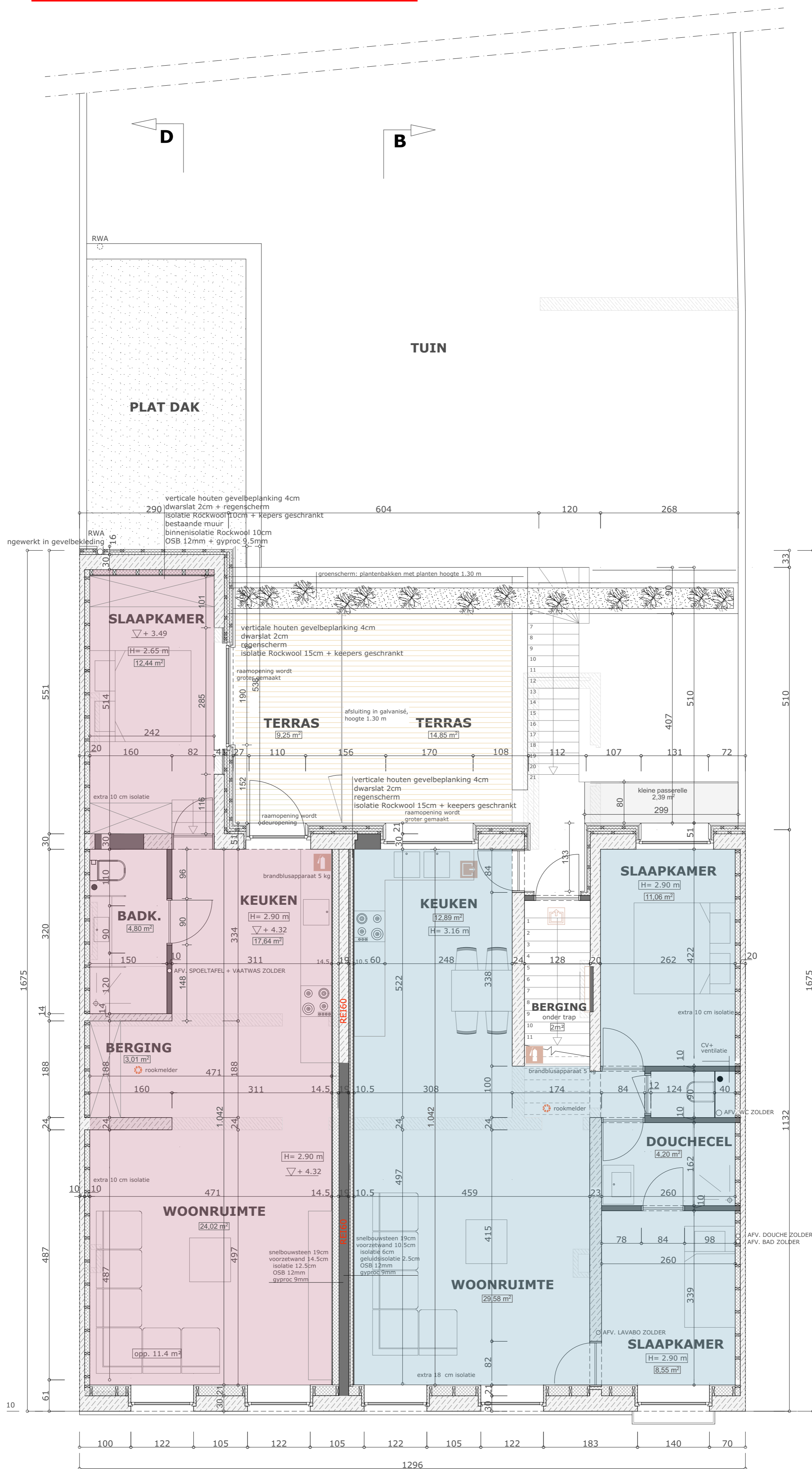
C A PLAN VERDIEPING nieuwe toestand - schaal 1:50
