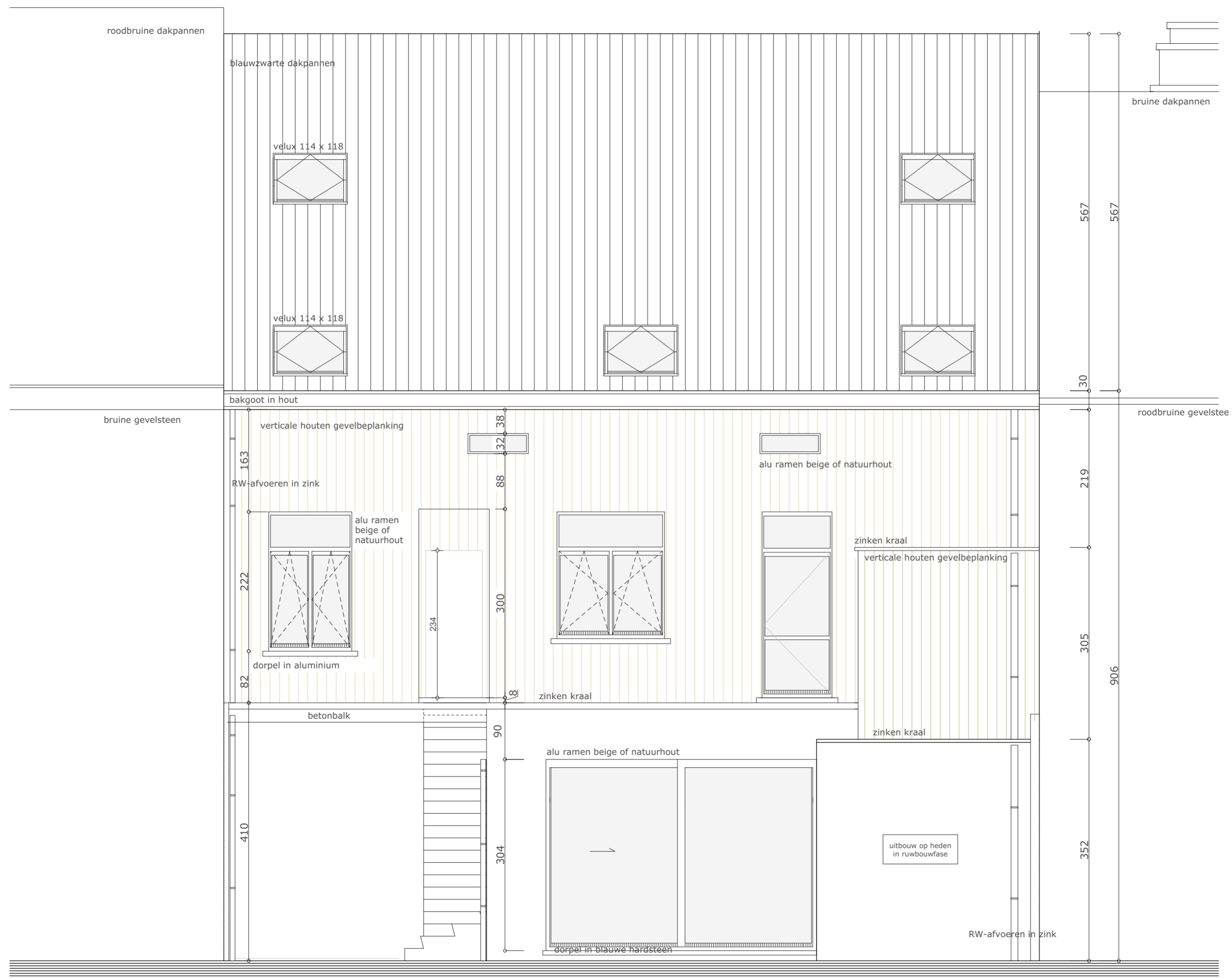
ACHTERGEVEL bestaande toestand - schaal 1:50
