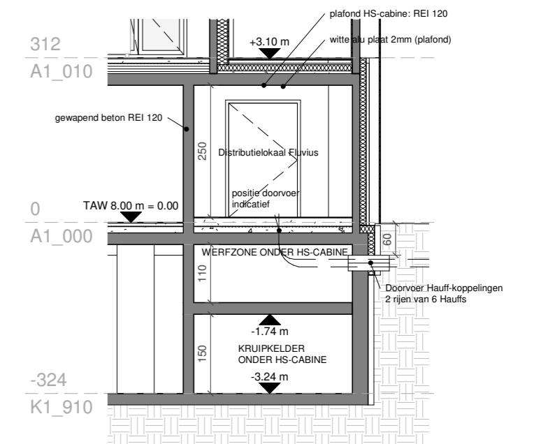
Principesnede GG distributielokaal Fluvius 1:100
