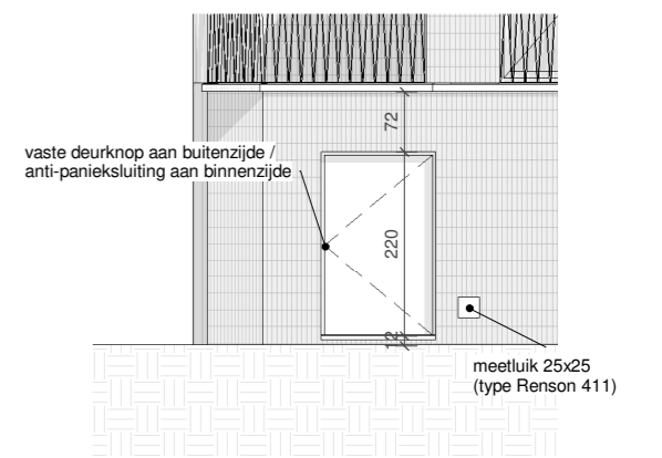
Noordoostgevel distributielokaal Fluvius 1:100
