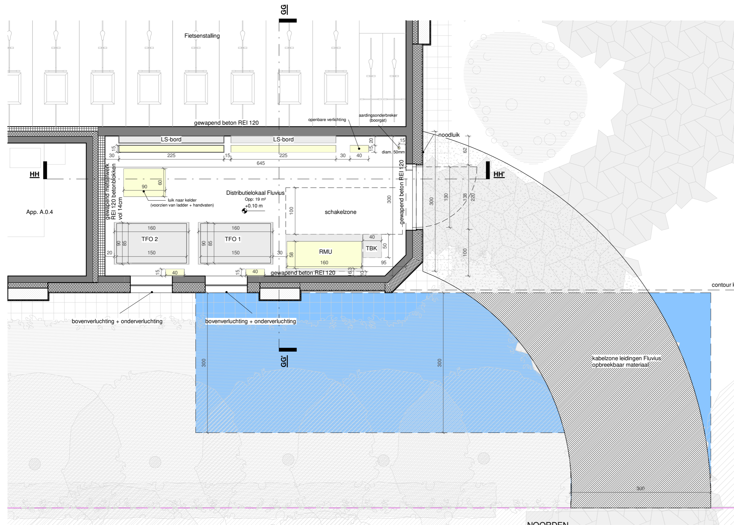
Grondplan distributielokaal Fluvius 1:50
