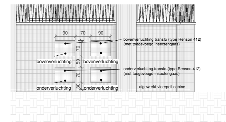
Zuidoostgevel distributielokaal Fluvius 1:100
