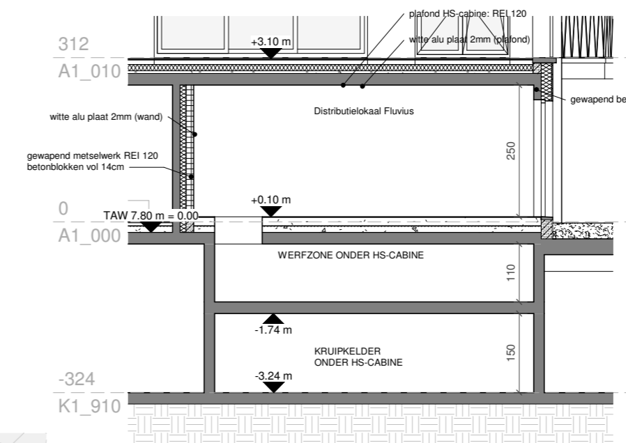
Principesnede HH distributielokaal Fluvius 1:100
