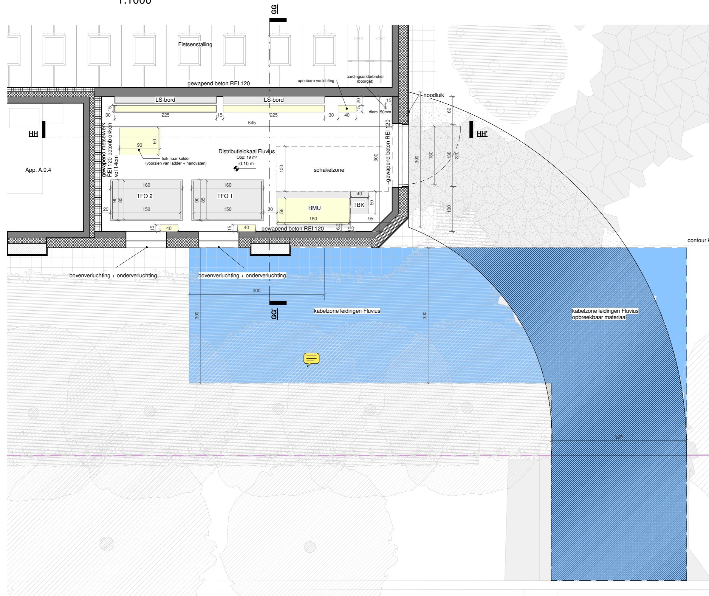
Grondplan distributielokaal Fluvius 1:50
