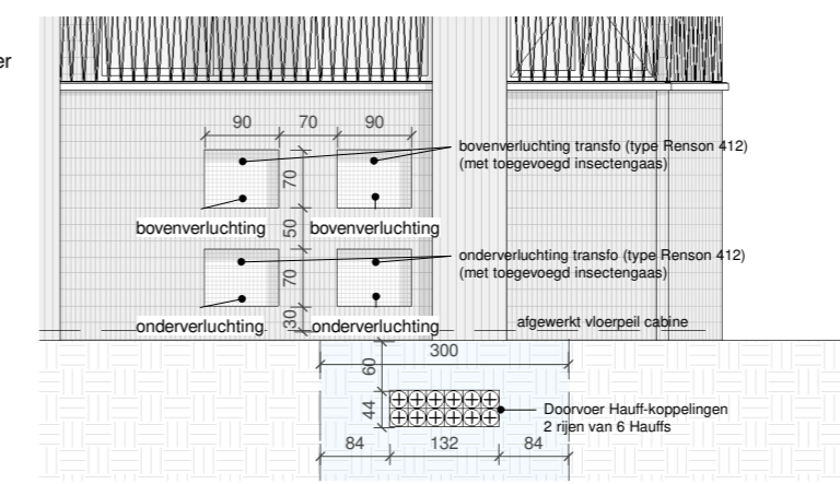
Zuidoostgevel distributielokaal Fluvius 1:100
