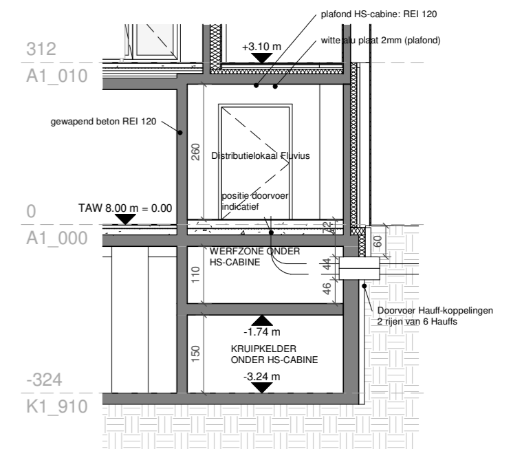
Principesnede GG distributielokaal Fluvius 1:100
