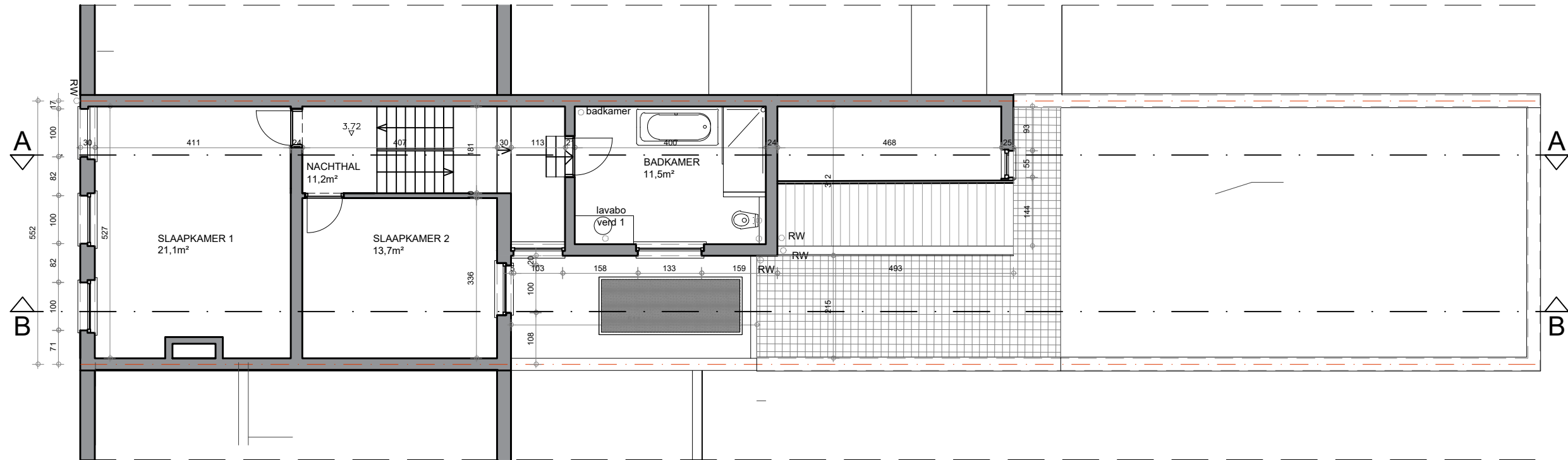
VERDIEPING 1 BESTAANDE TOESTAND
