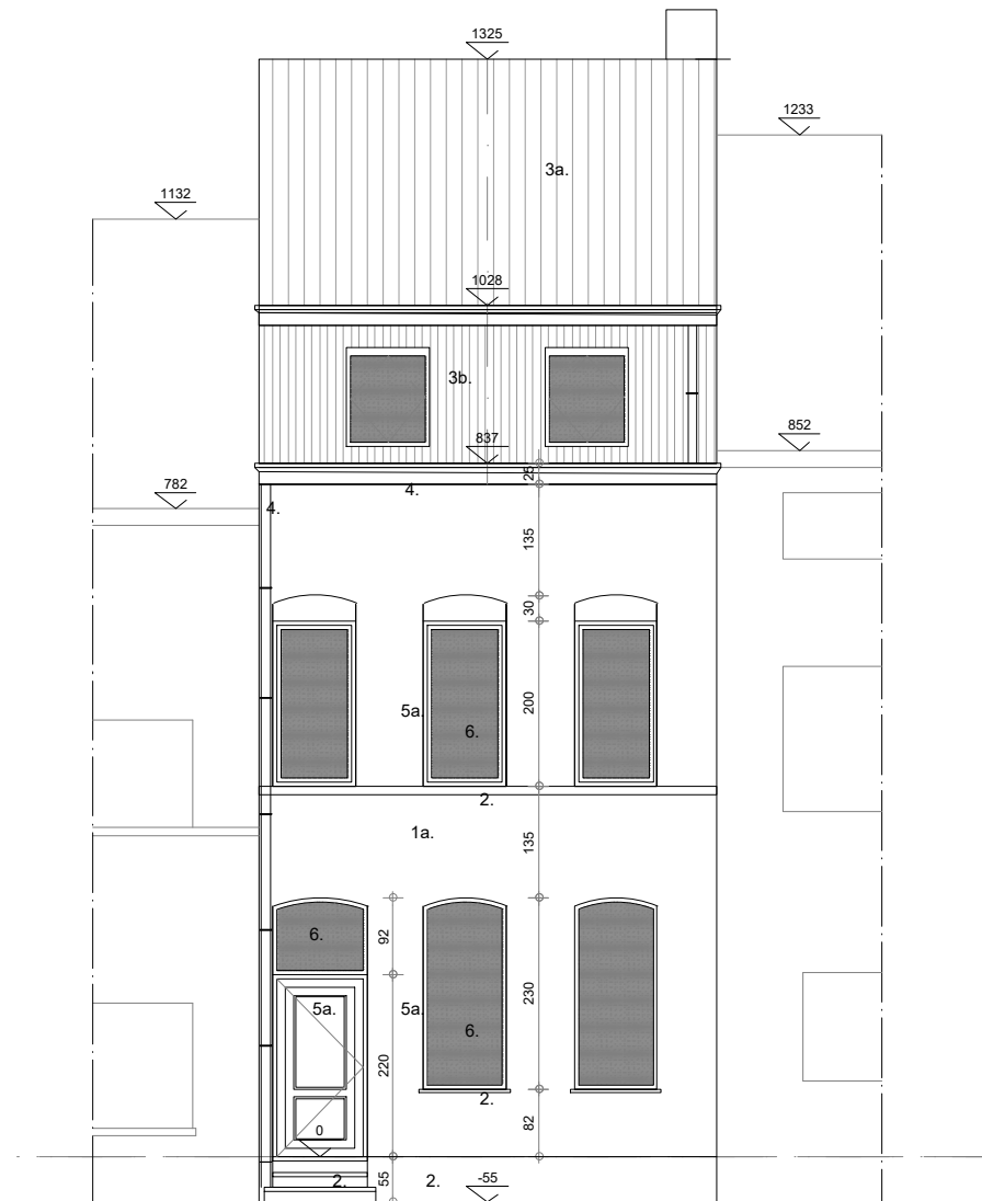
VOORGEVEL NIEUWE TOESTAND
