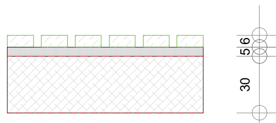
principesnede. | waterdoorlatende klinkers (helling max. 2%)
