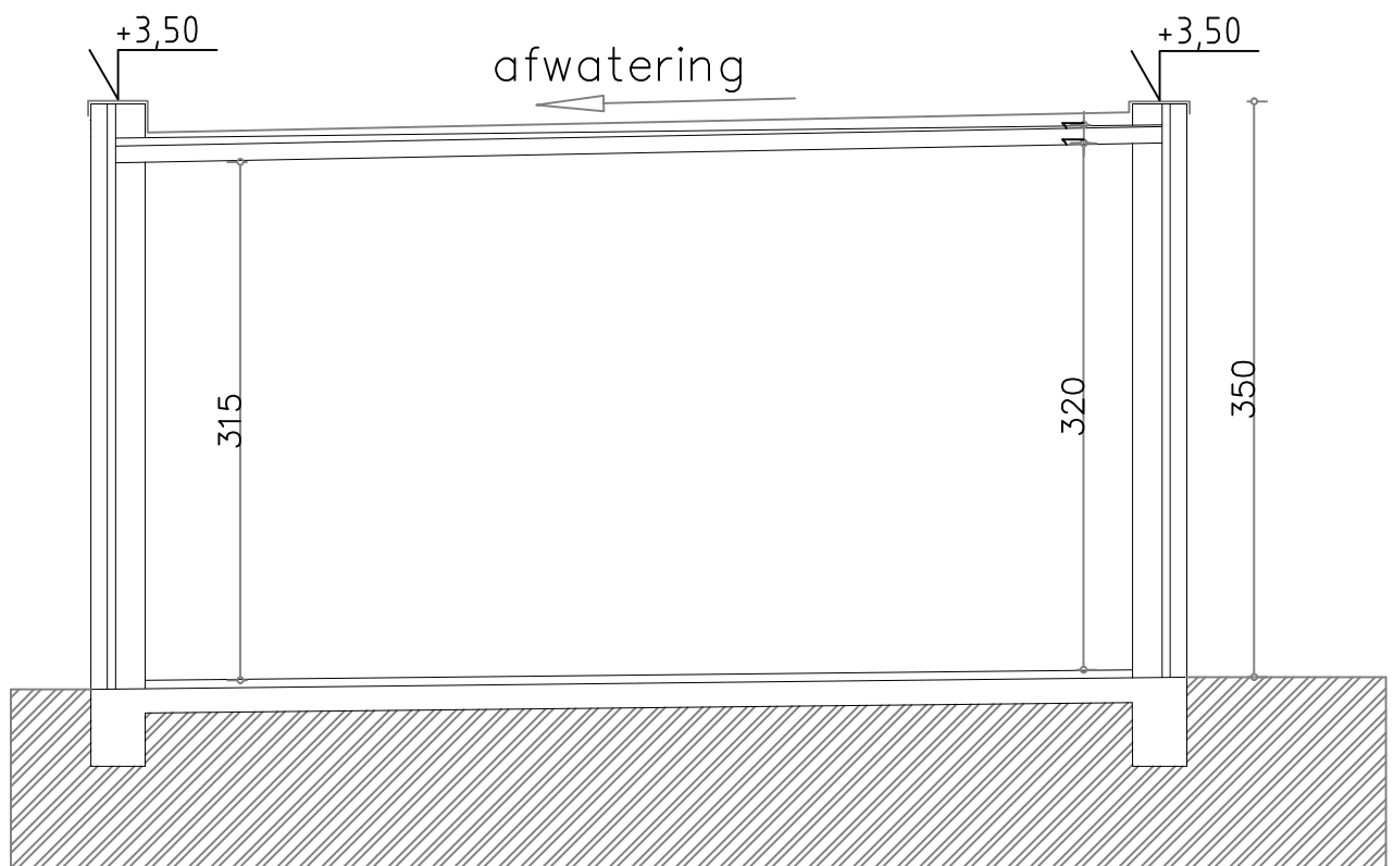
Nieuwe toestand Doorsnede schaal 1/50
