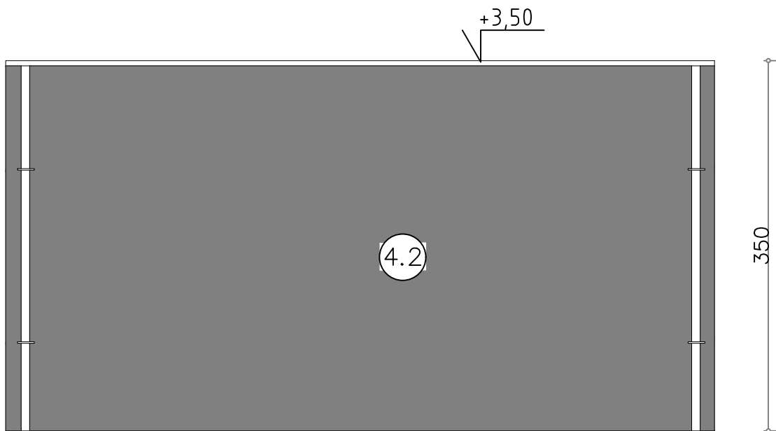
Nieuwe toestand Gevel links schaal 1/50
