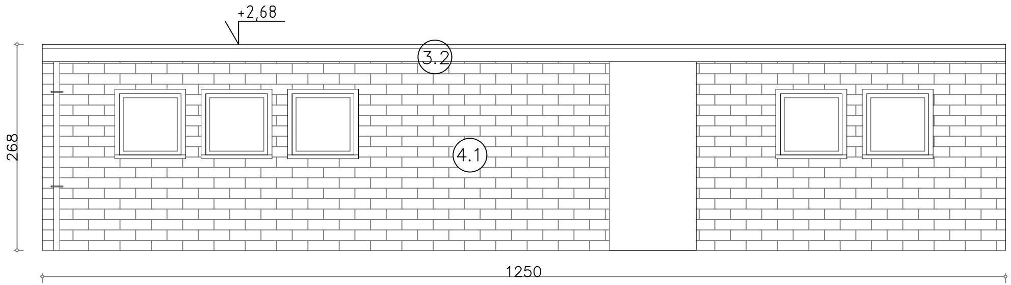
Bestaande toestand Gevel rechts schaal 1/50
