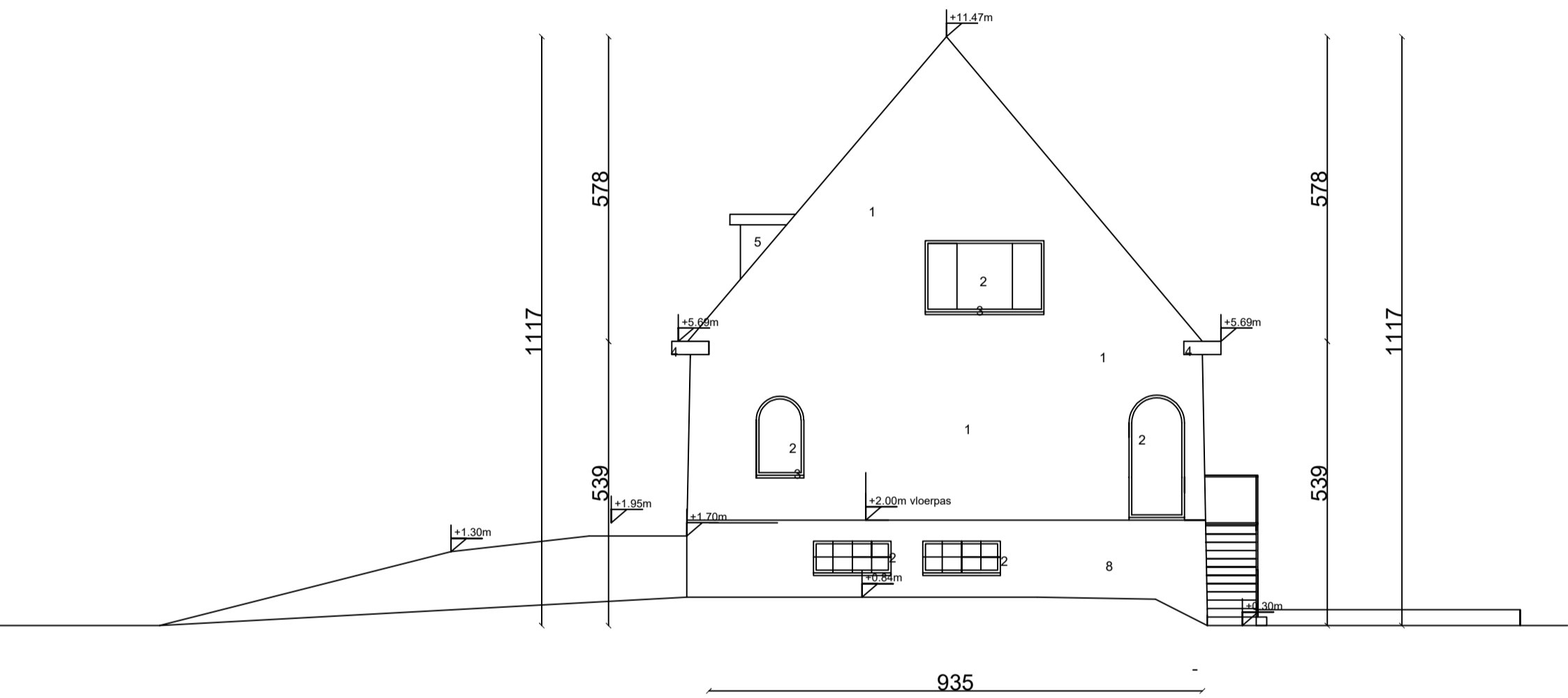
RECHTERZIJGEVEL 1/100 Bestaande toestand
